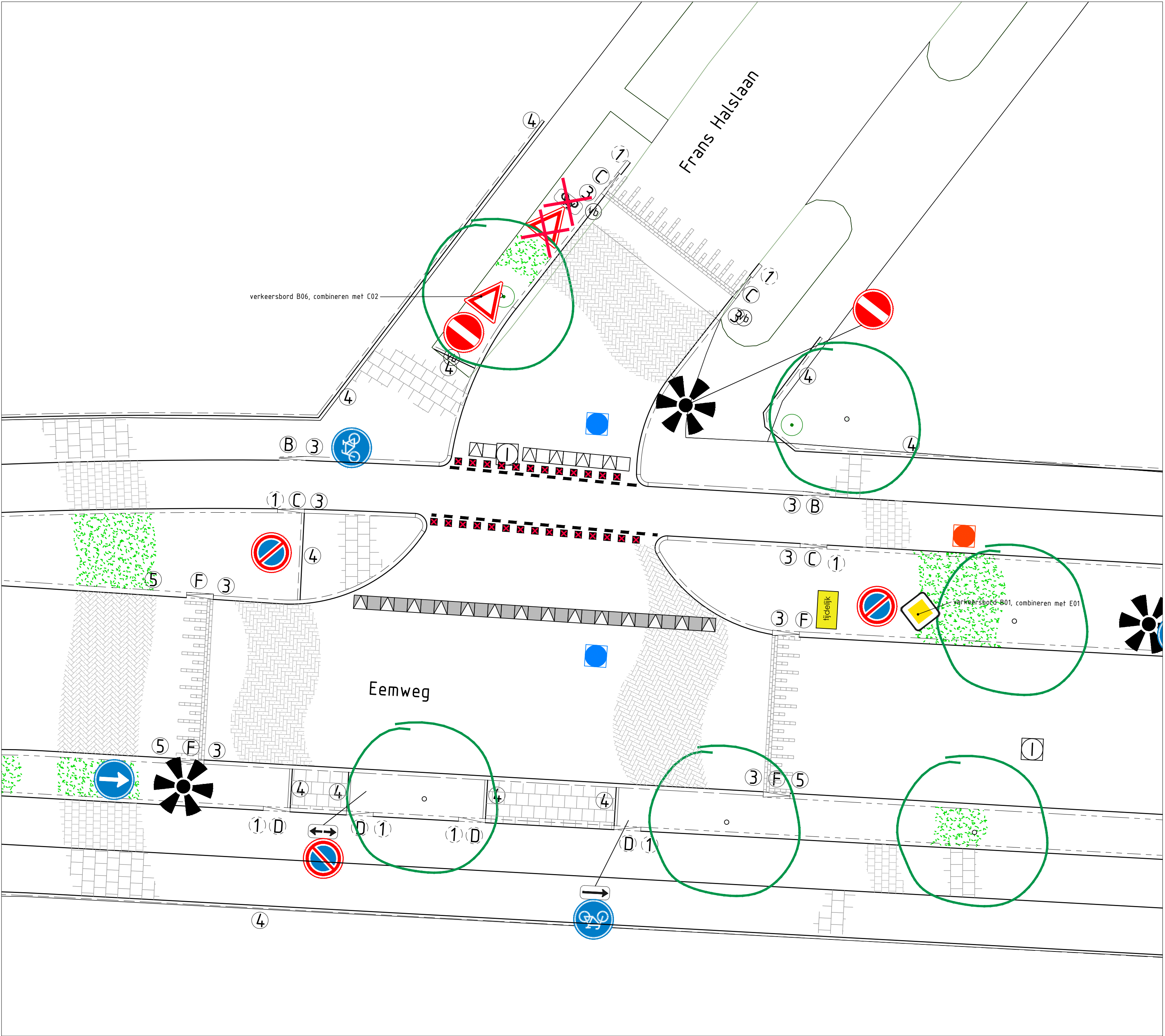
Plansituatie kruispunt Eemweg - Frans Halslaan Schaal : 1:100
