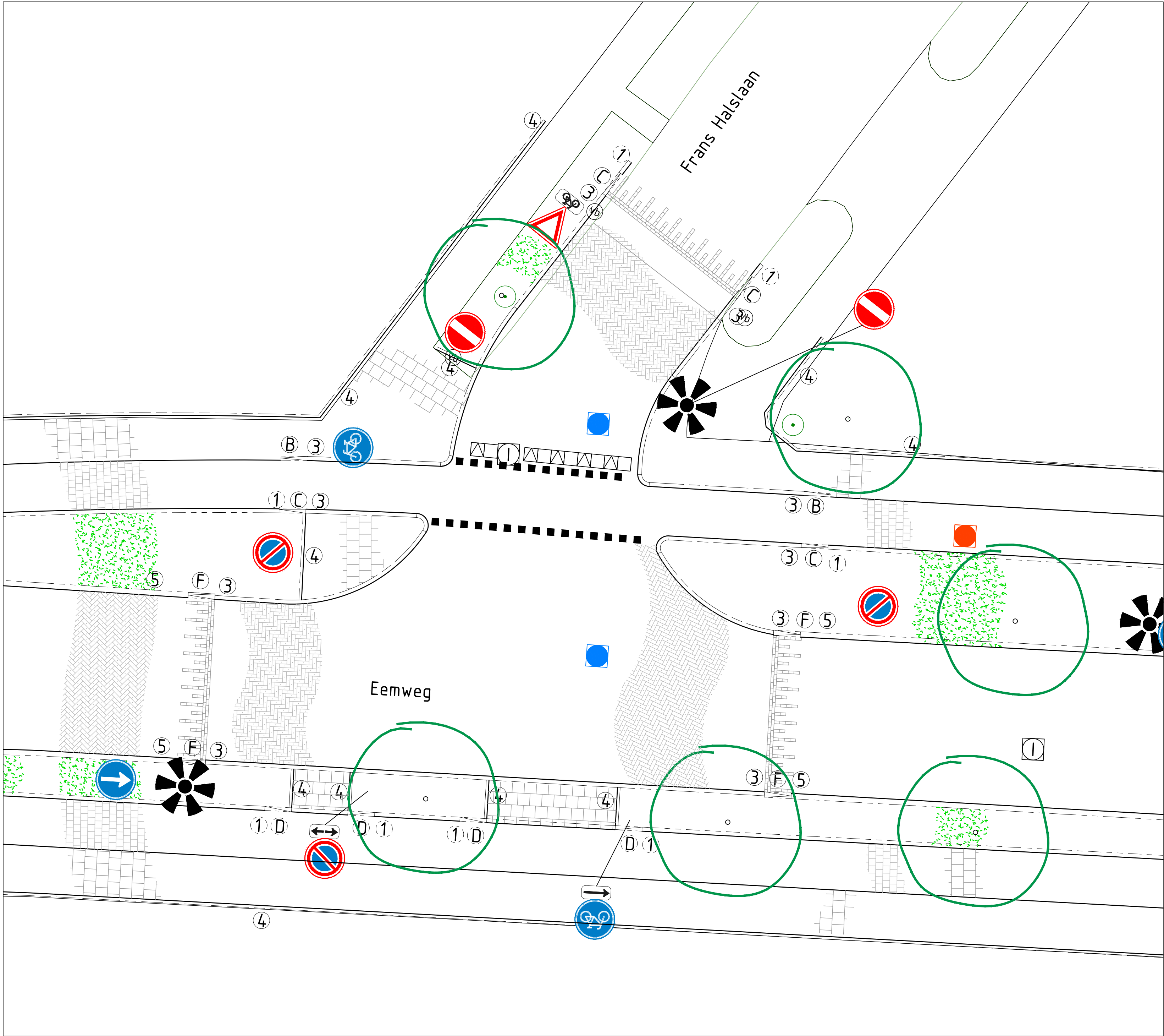
Bestaande situatie kruispunt Eemweg - Frans Halslaan Schaal : 1:100
