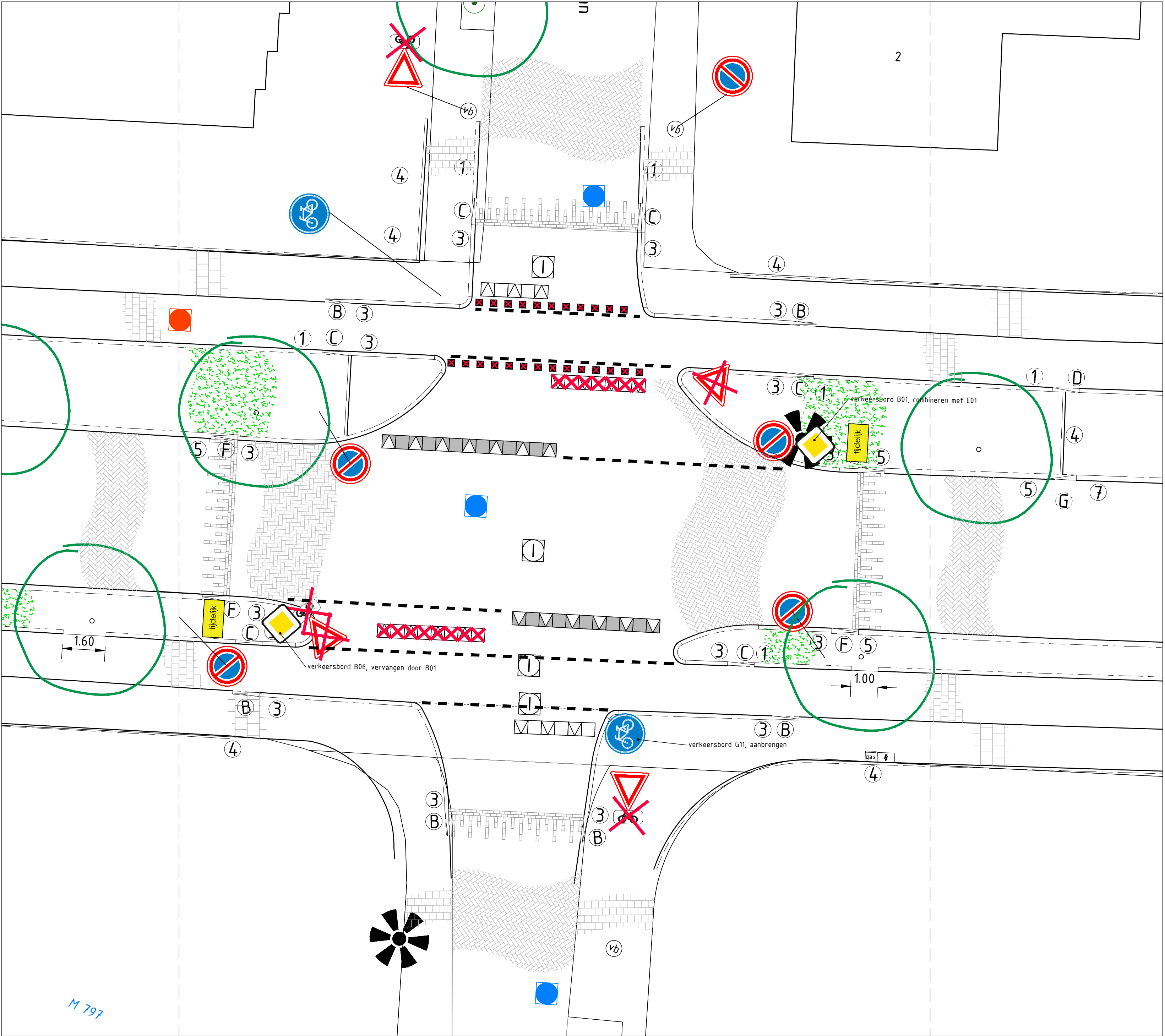
Plansituatie kruispunt Eemweg - Rembrandtlaan - Tromplaan Schaal : 1:100
