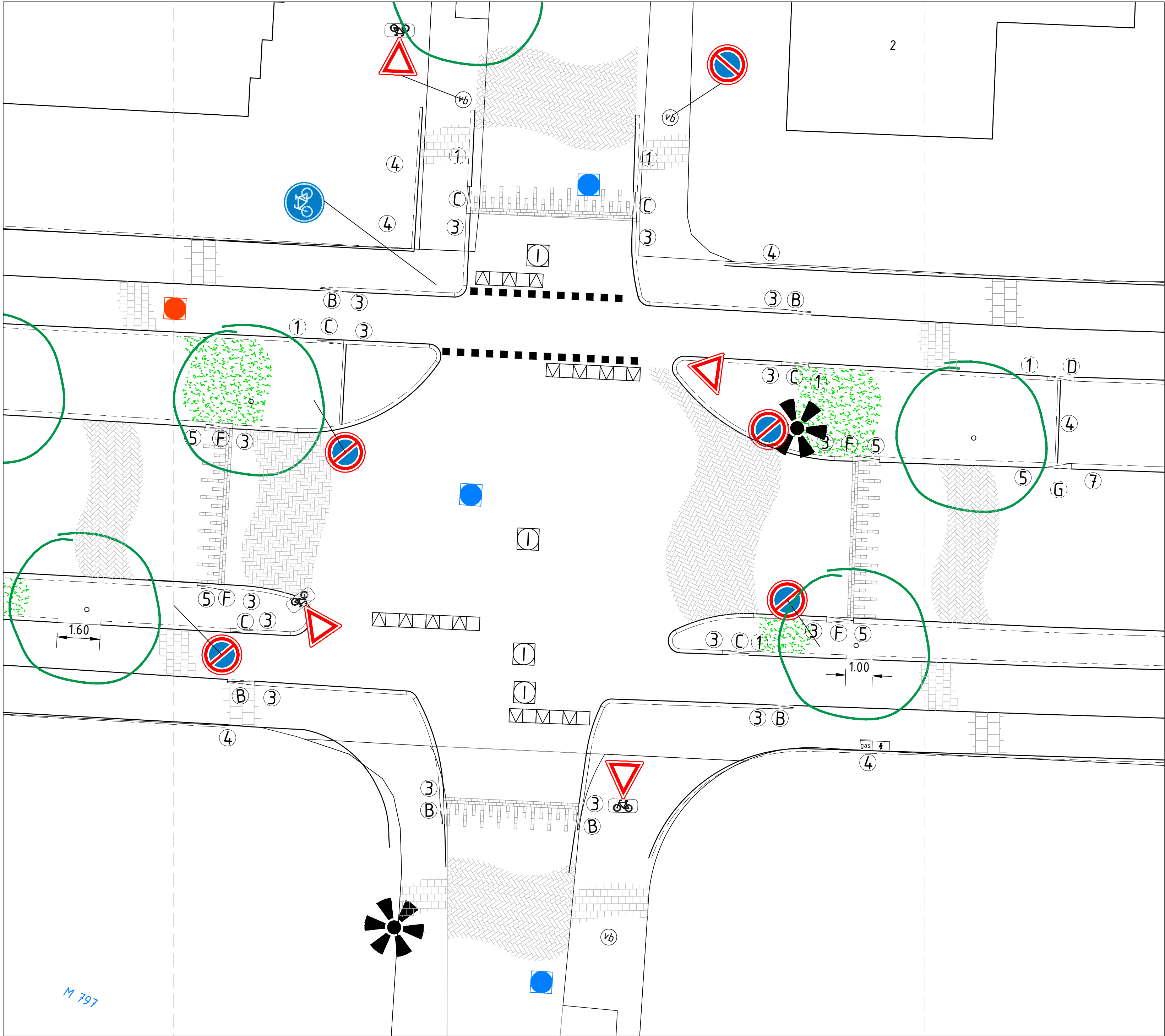
Bestaande situatie kruispunt Eemweg - Rembrandtlaan - Tromplaan Schaal : 1:100
