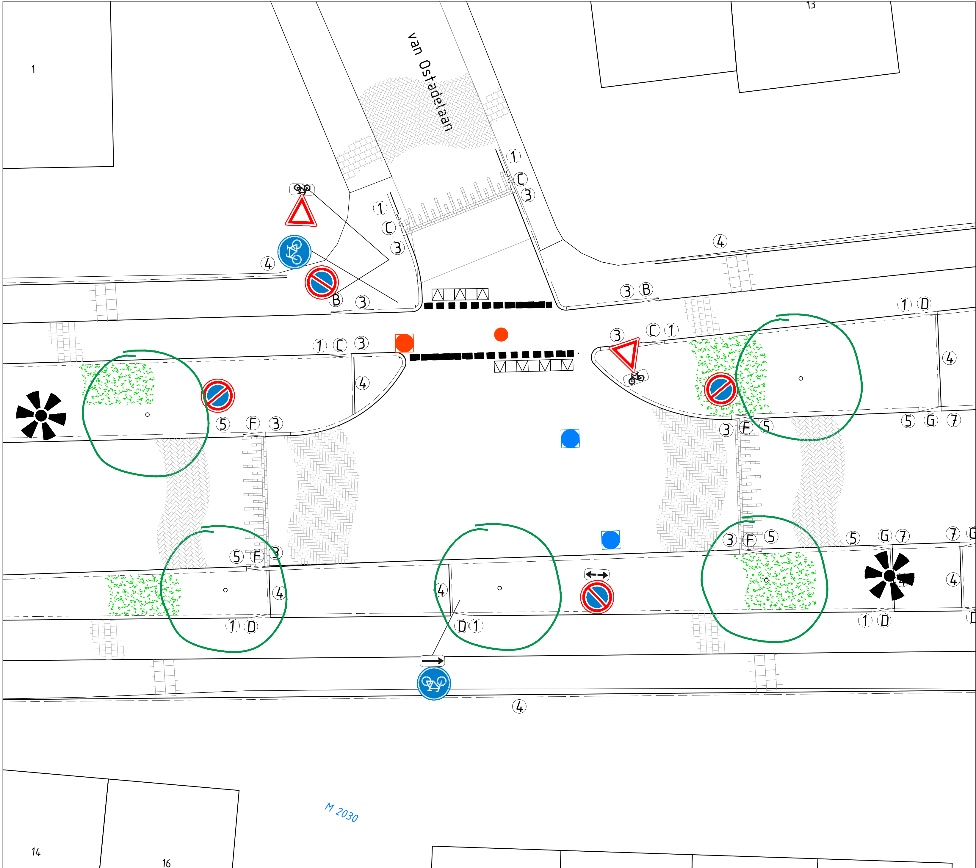
Bestaande situatie kruispunt Eemweg - van Ostadelaan Schaal : 1:100
