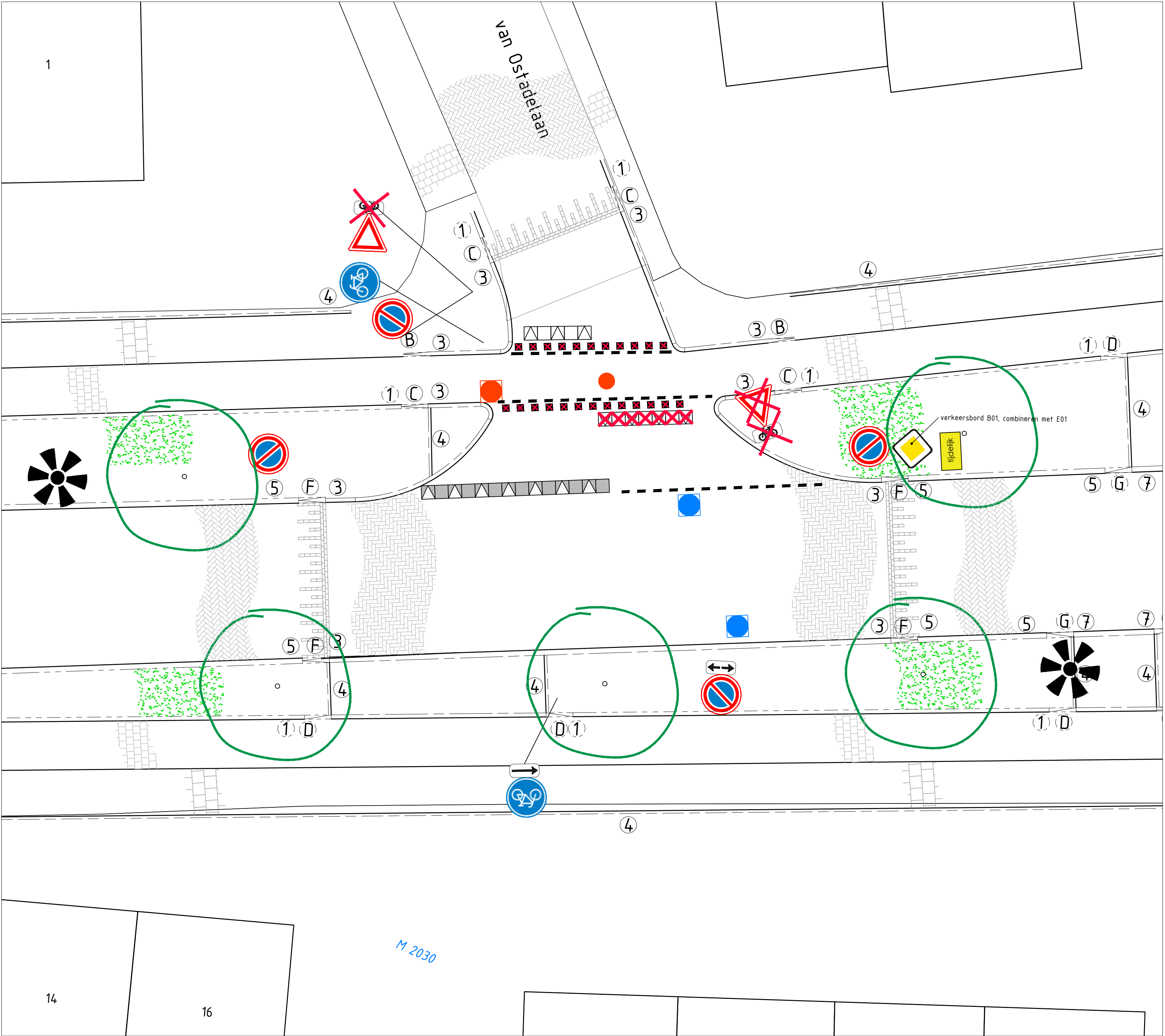
Plansituatie kruispunt Eemweg - van Ostadelaan Schaal : 1:100
