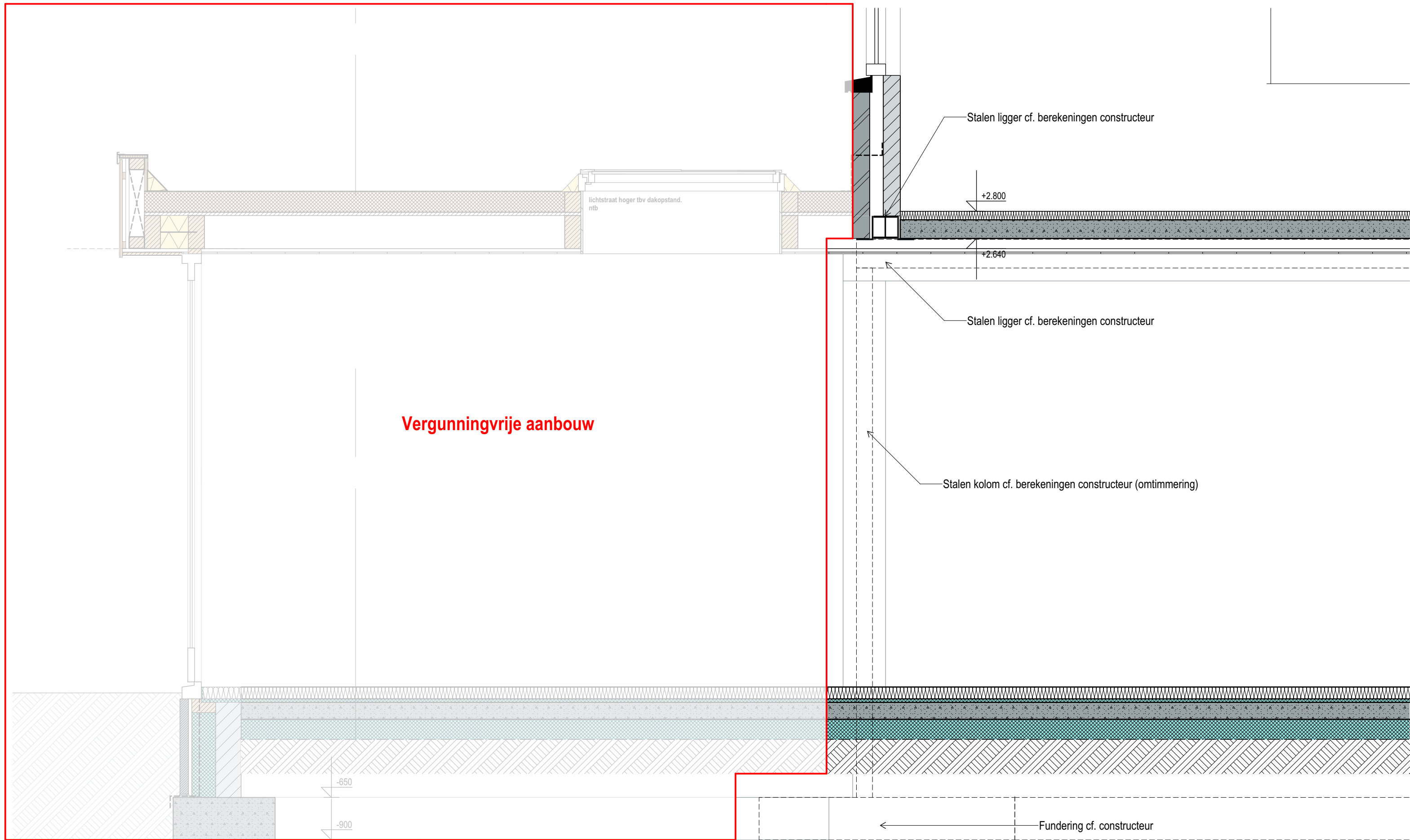
A Doorsnede A 1:20
