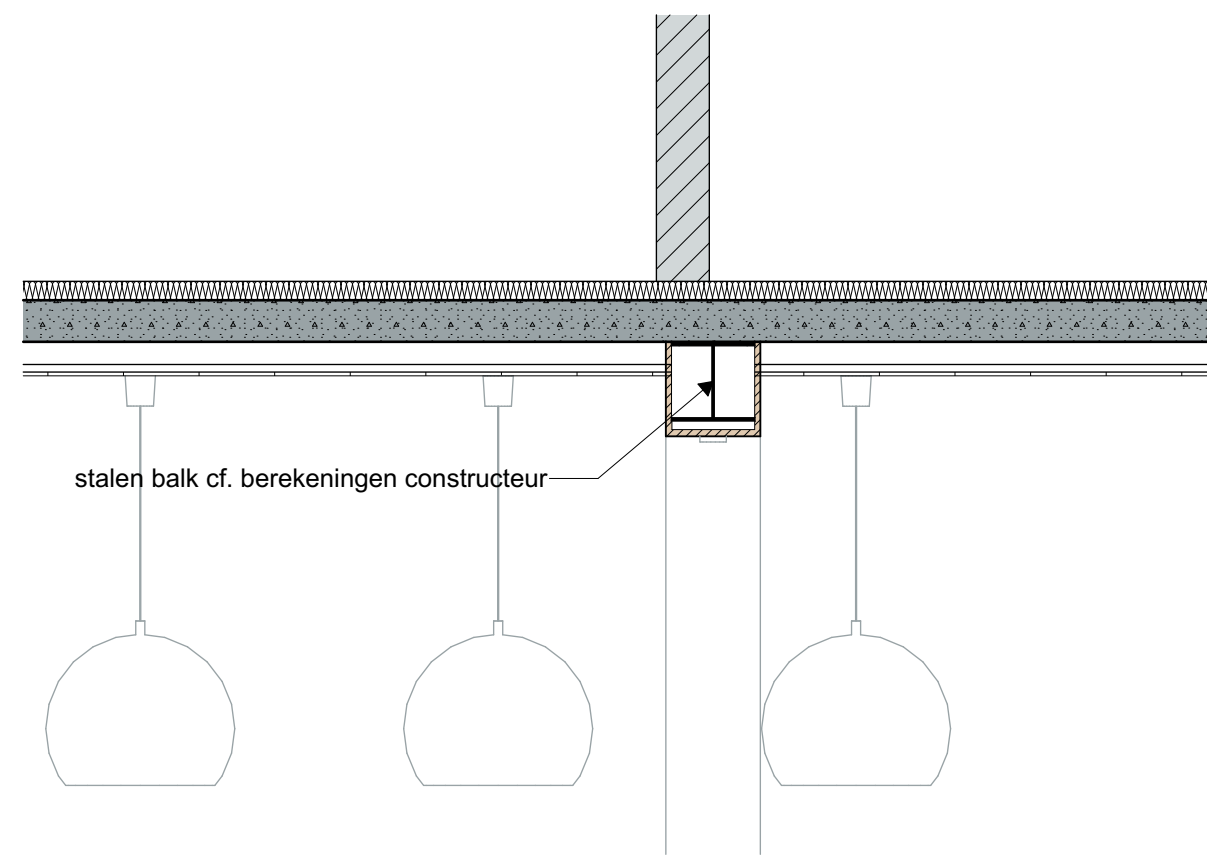
D Doorsnede D 1:20
