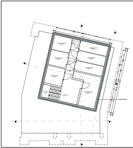
afb. 8 Kelder
