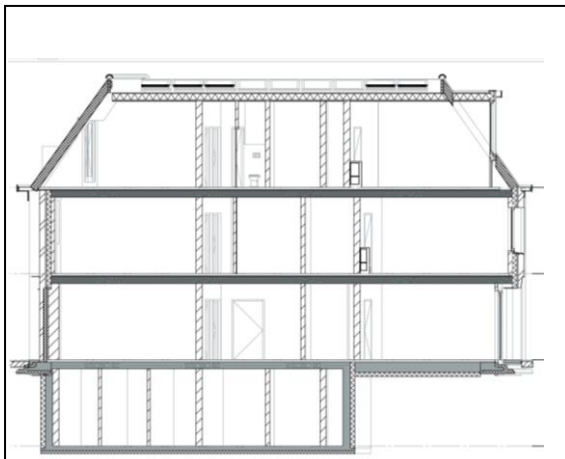
afb. 12 Langsdoorsnede
