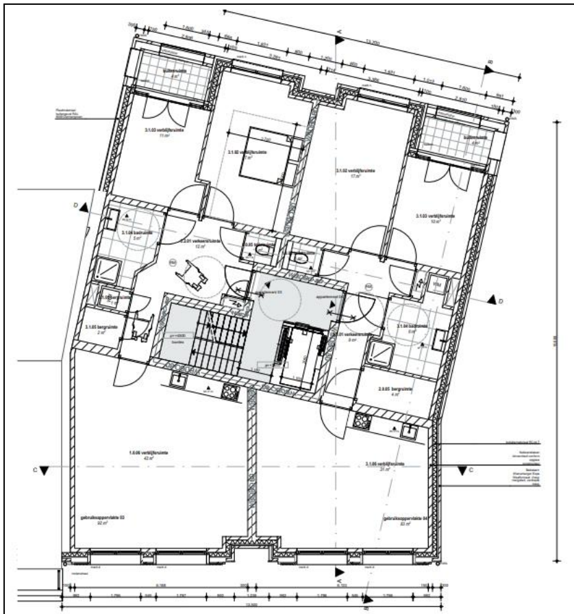
afb. 6 Plattegrond 1 e verdieping
