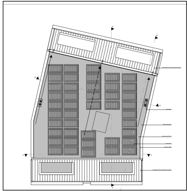
afb. 9 Dakaanzicht met zonnepanelen
