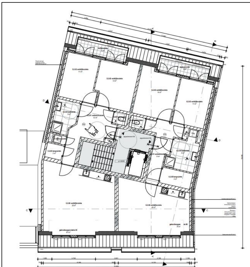
afb. 7 Plattegrond 2 e verdieping
