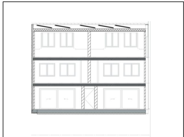
afb. 13 Dwarsdoorsnede
