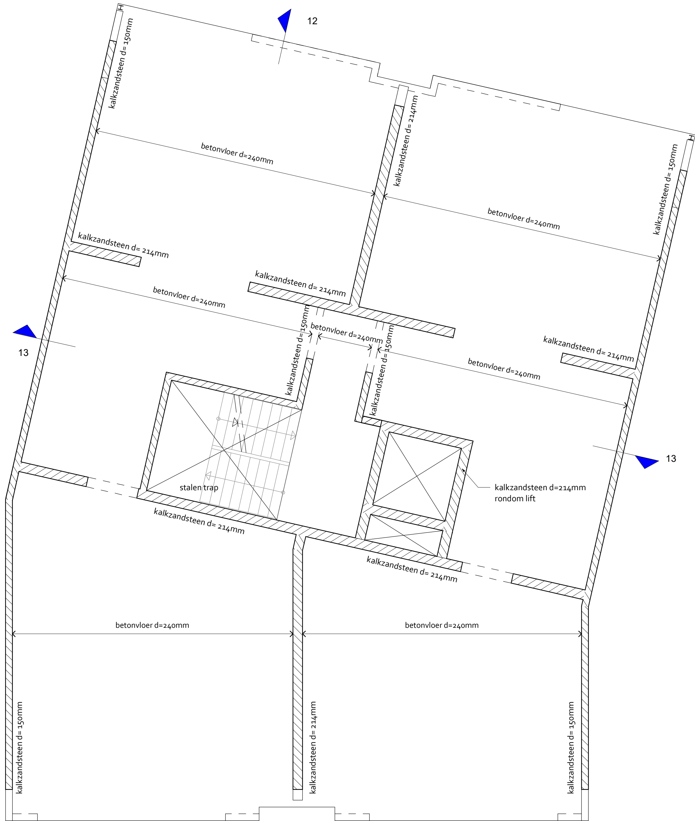
2e verdiegingsvloer 1 : 50
