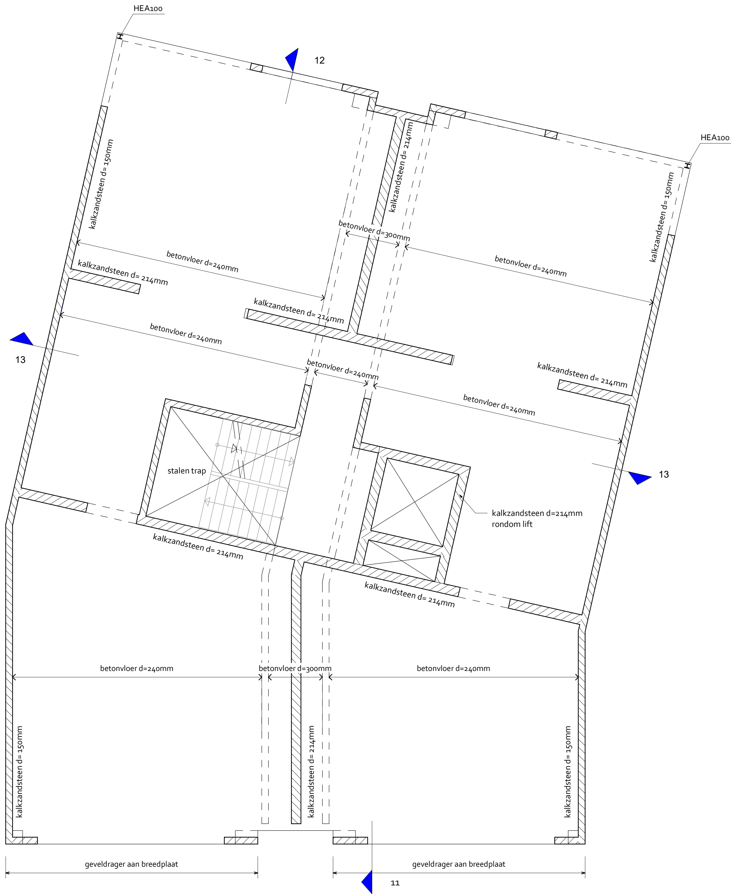
1e verdiegingsvloer 1 : 50
