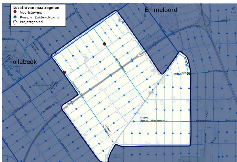
Figuur 1: projectgebied met locatie voortstuwers (rode stippen) en pompinstallatie (blauwe stip)
