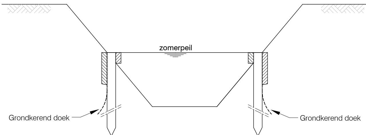
Dwarsdoorsnede
