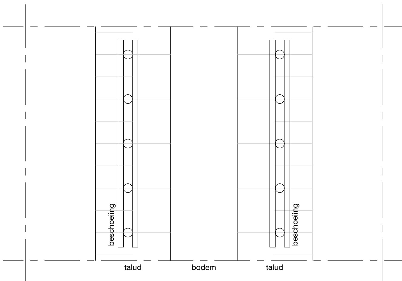
Bovenaanzicht
