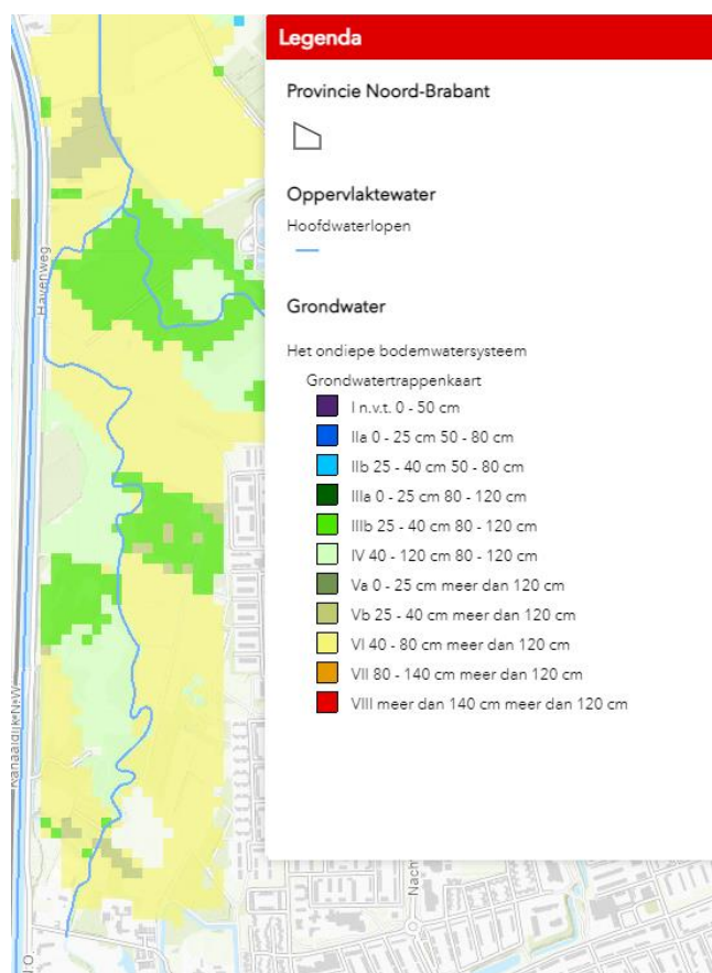
Figuur 5: Grondwatertrappen
