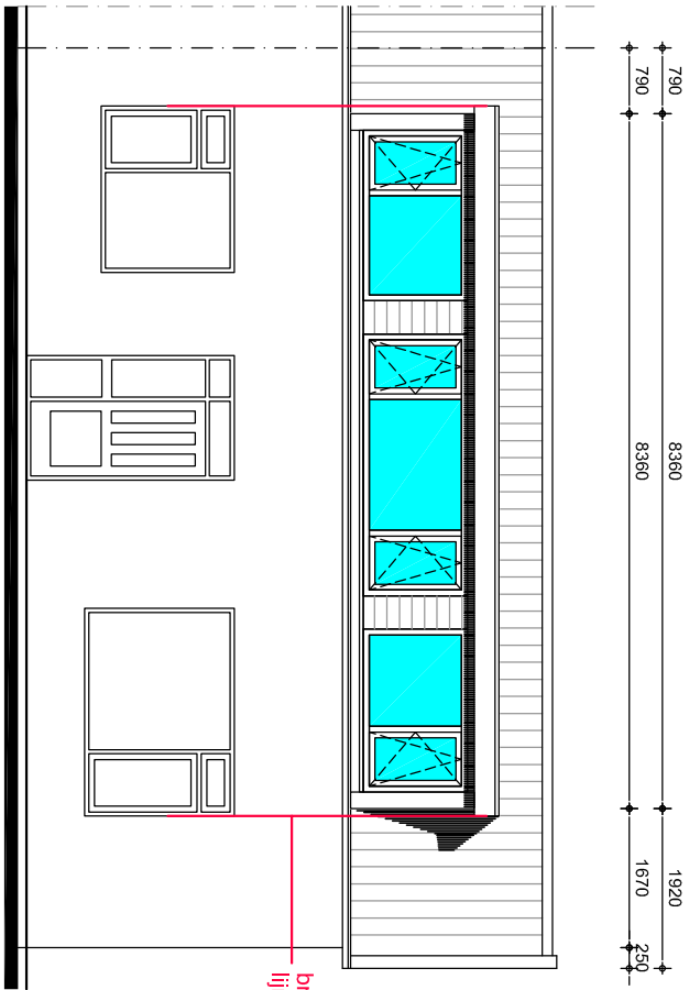
= Voorgevel nieuw =
