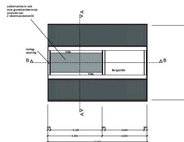
- 1E VERDIEPING -
