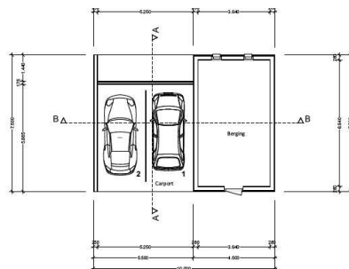
- BEGANE GROND -
