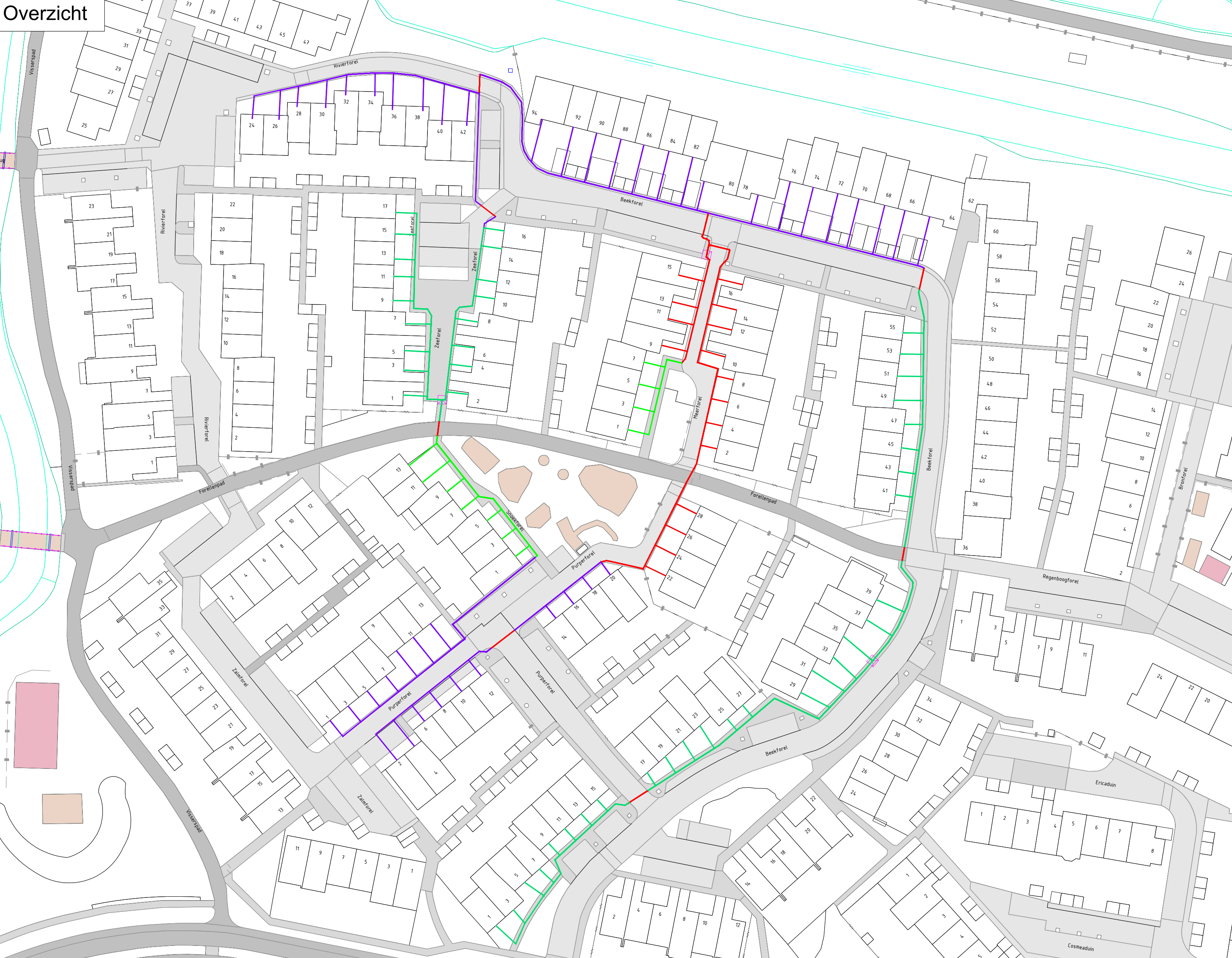
Detail 2, voetpad afsluiten CROW 96b fig.1103a
