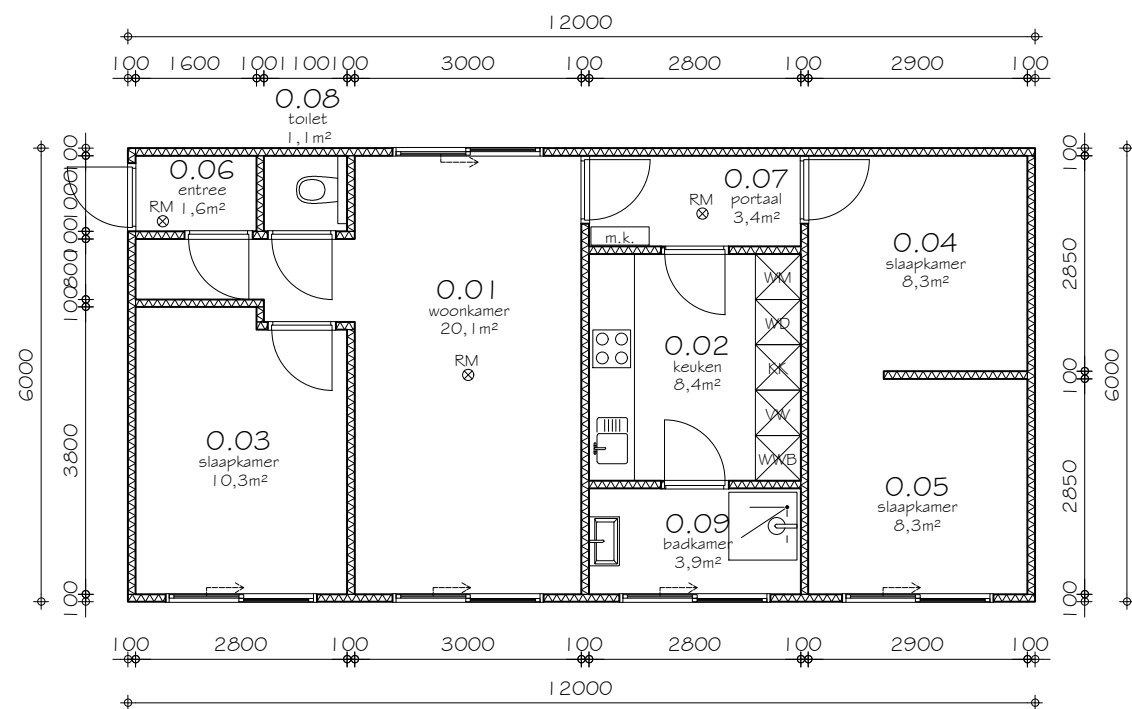
PLATTEGROND
