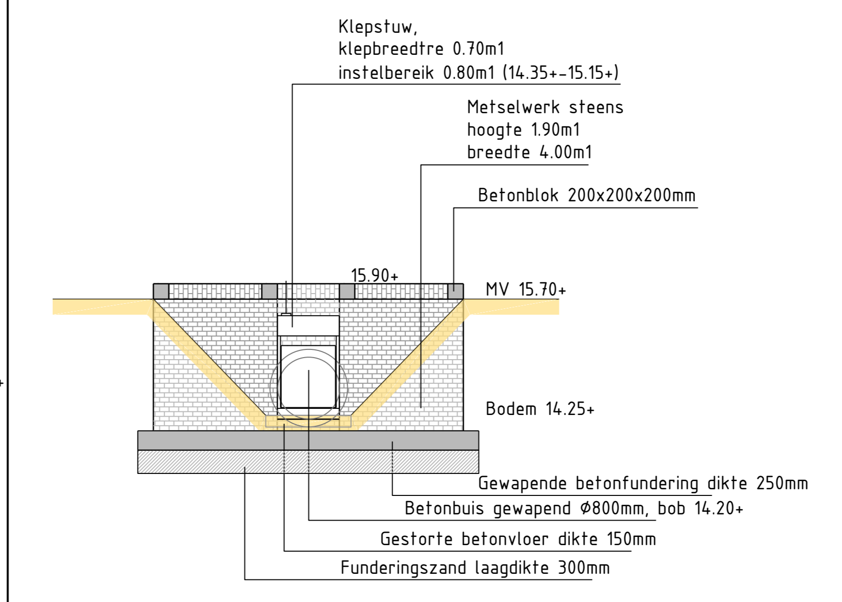
Aanzicht duiker met klepstuw Schaal 150
