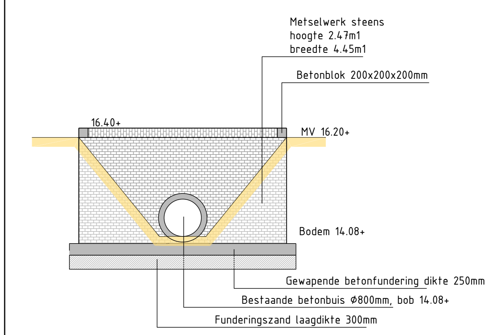
Aanzicht muur duiker weg Schaal 150
