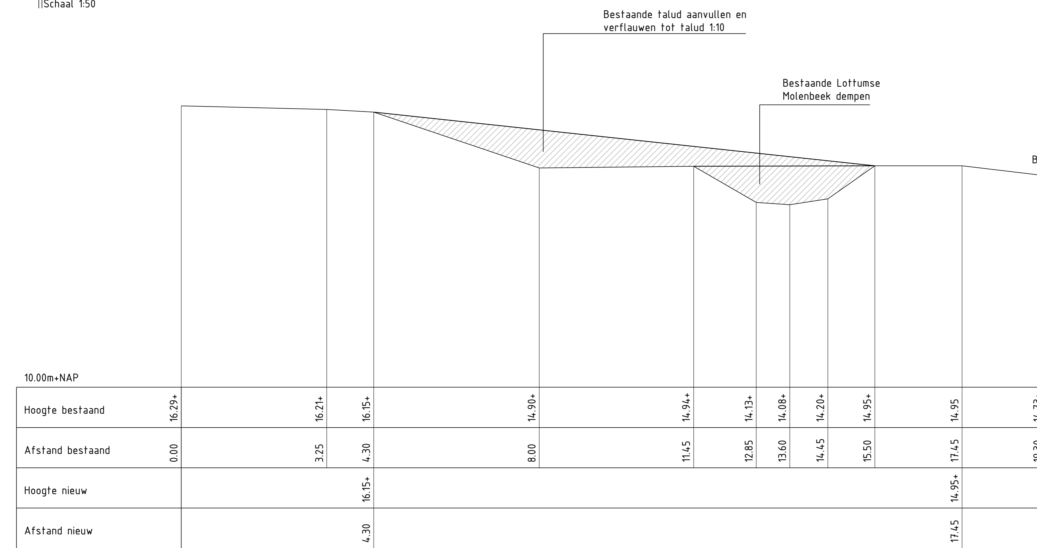
Dwarsprofiel B Schaal 1:50
