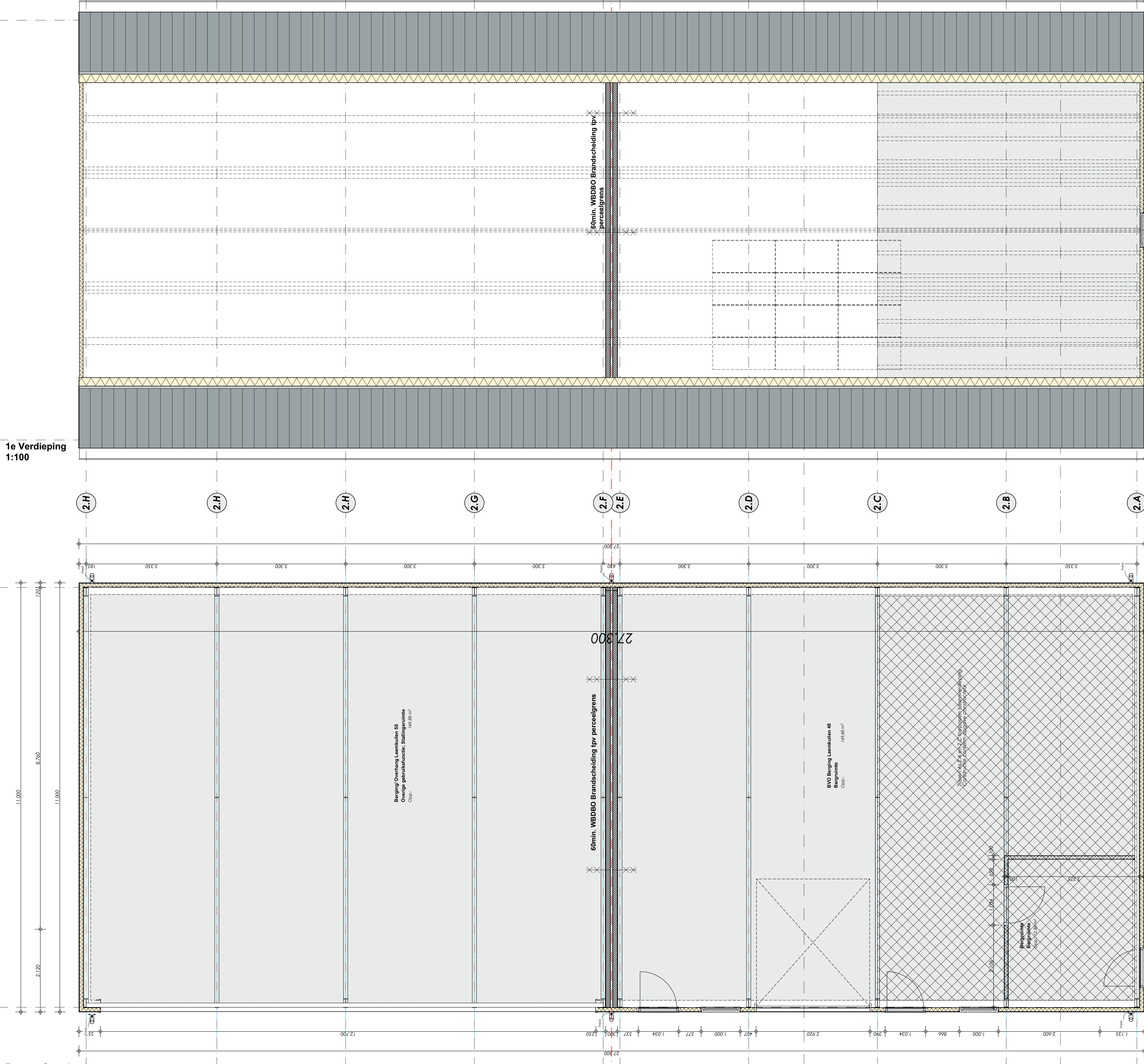
Begane Grond 1:100
