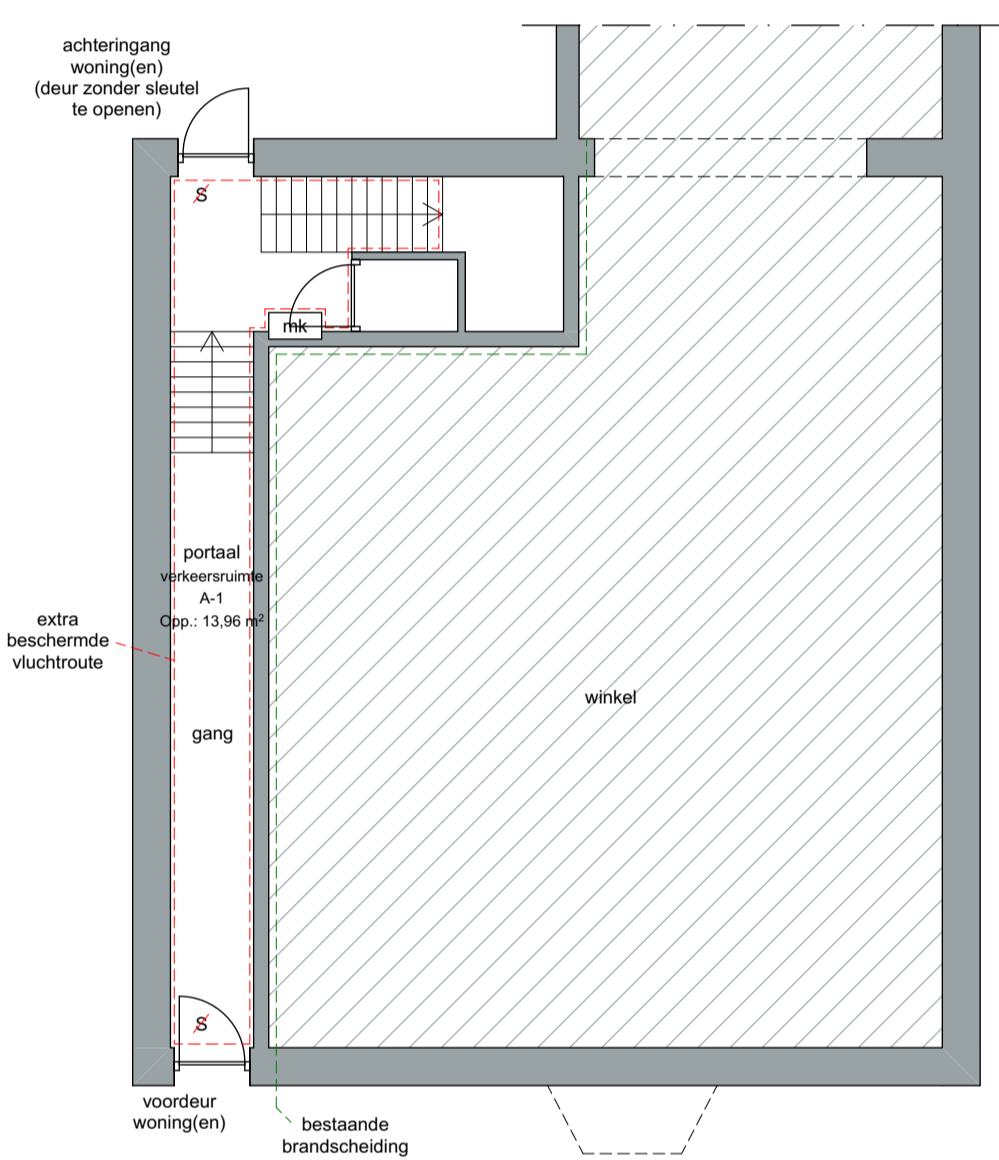
begane grond bestaand / NIEUW
