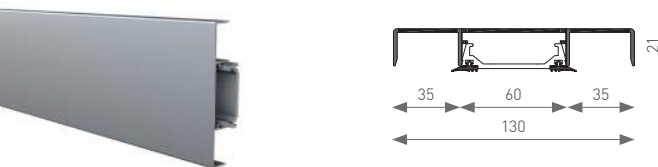
HF4 - DECORATIEF OMEGA-PROFIEL
