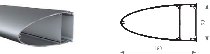
HF8 - ELLIPTISCH DECORATIEF PROFIEL
