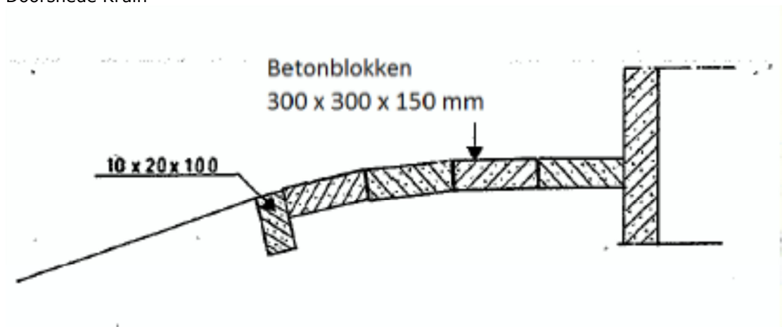
Detail constructie
