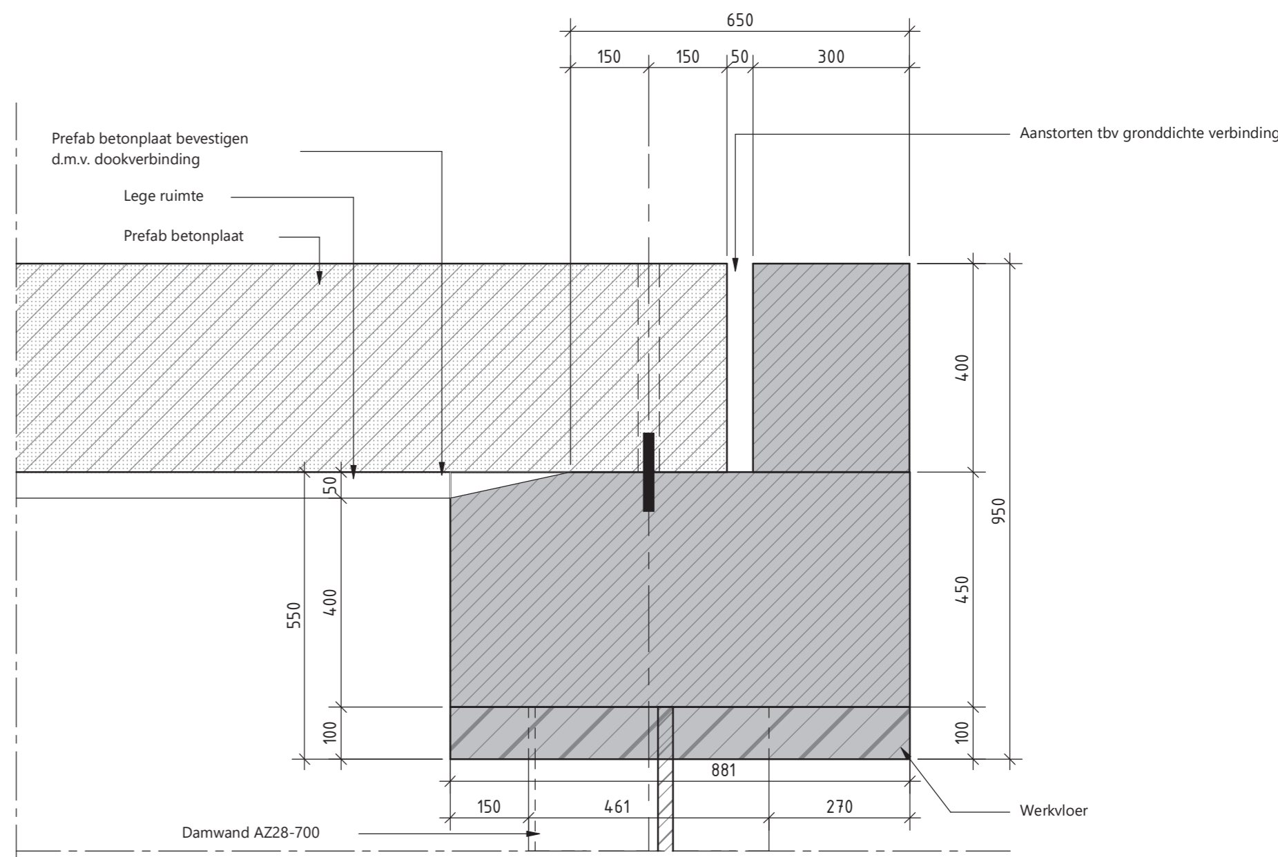
DETAIL OPLEGGING schaal: 1:10
