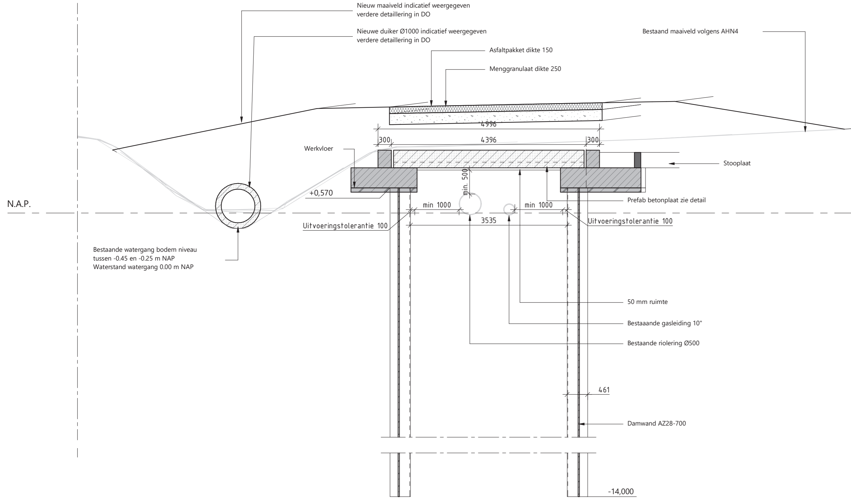
DWARSDOORSNEDE A-A schaal: 1:50
