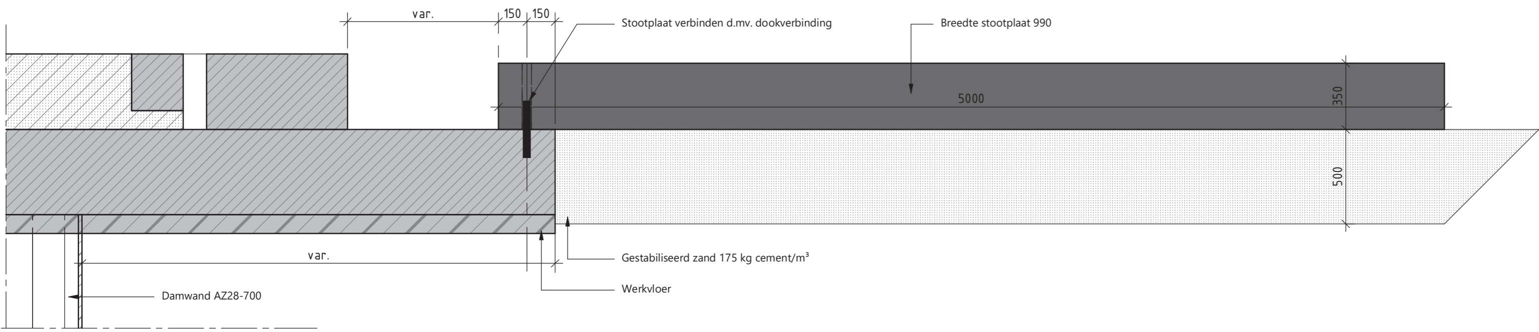
DWARSDOORSNEDE C-C schaal: 1:20
