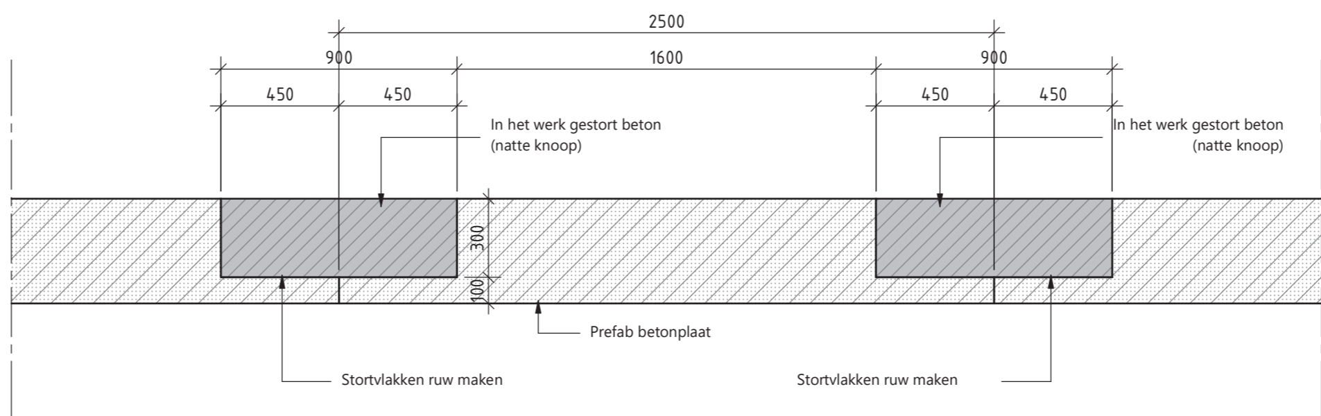
DWARSDOORSNEDE PREFAB BETONPLAAT (NATTE KNOOP) schaal: 1:20
