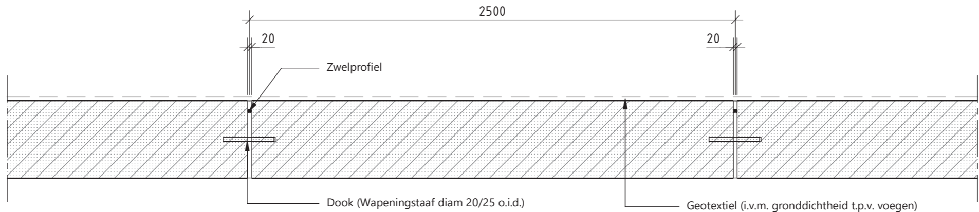
DWARSDOORSNEDE PREFAB BETONPLAAT schaal: 1:20
