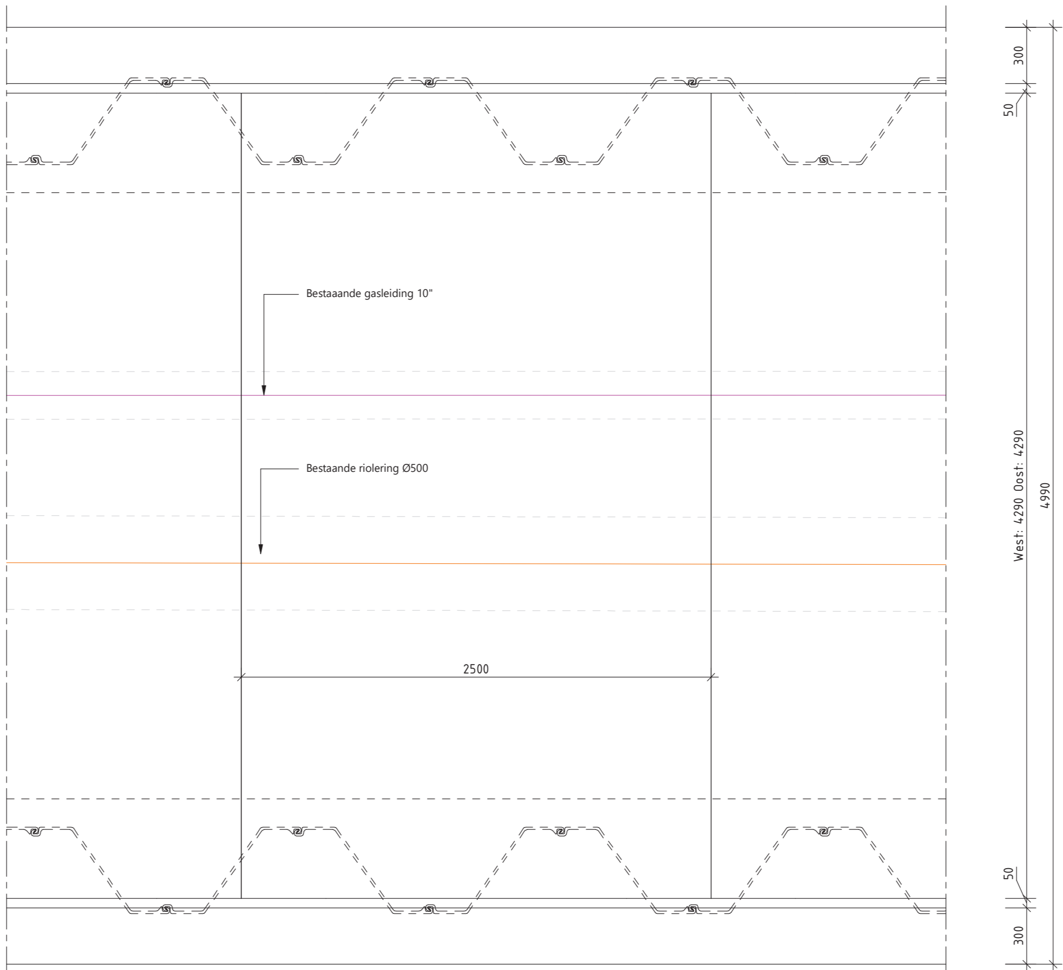
BOVENAANZICHT PREFAB BETONPLAAT schaal: 1:20
