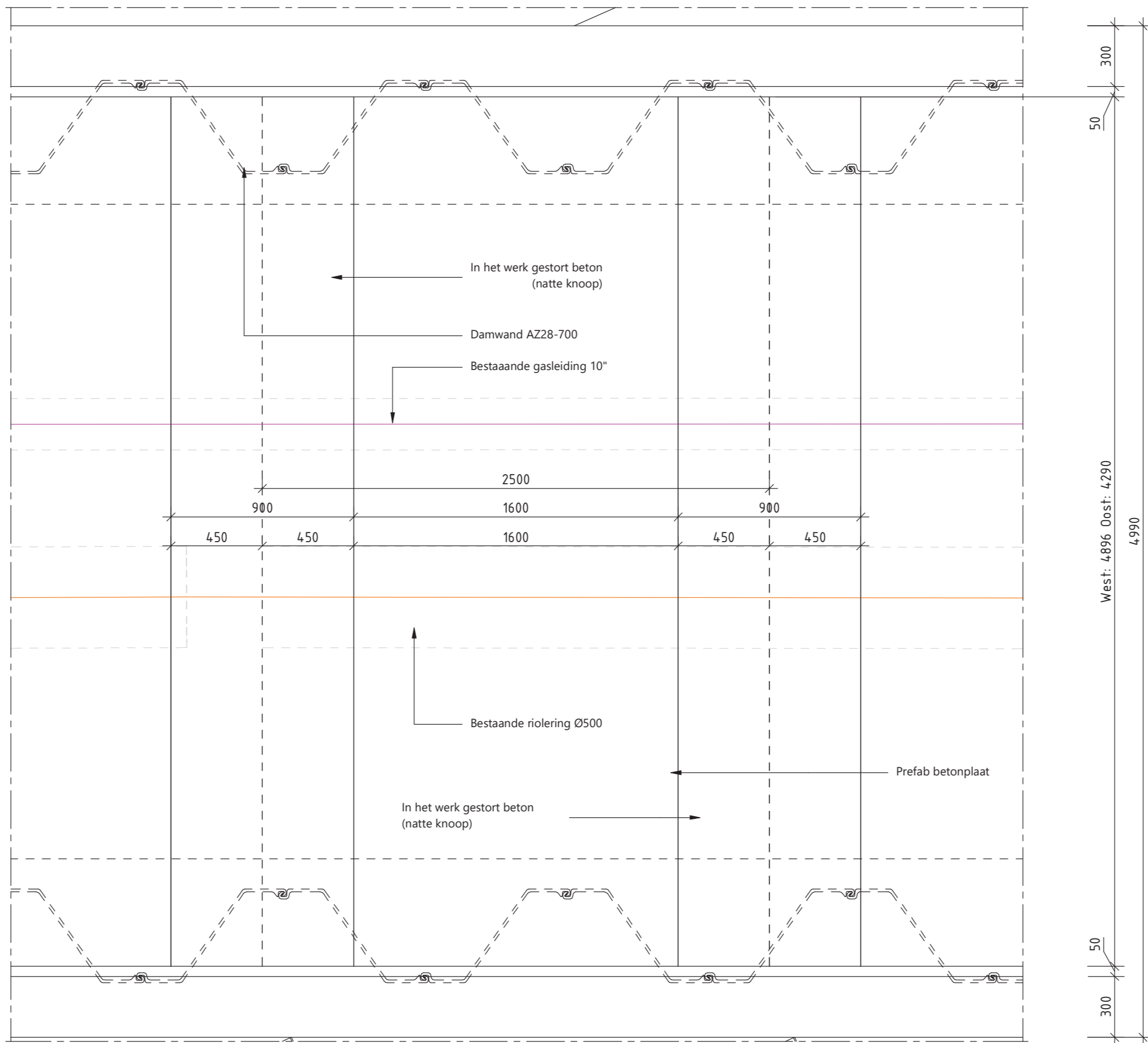
BOVENAANZICHT PREFAB BETONPLAAT (NATTE KNOOP) schaal: 1:20
