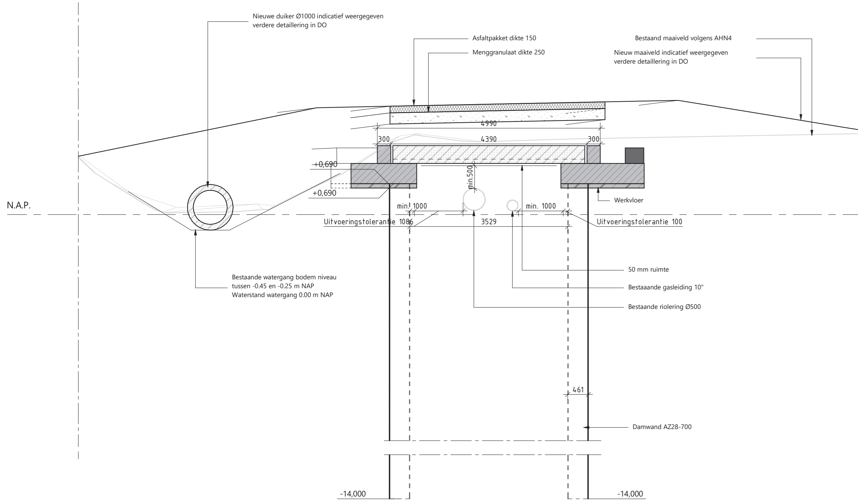
DWARSDOORSNEDE B-B schaal: 1:50
