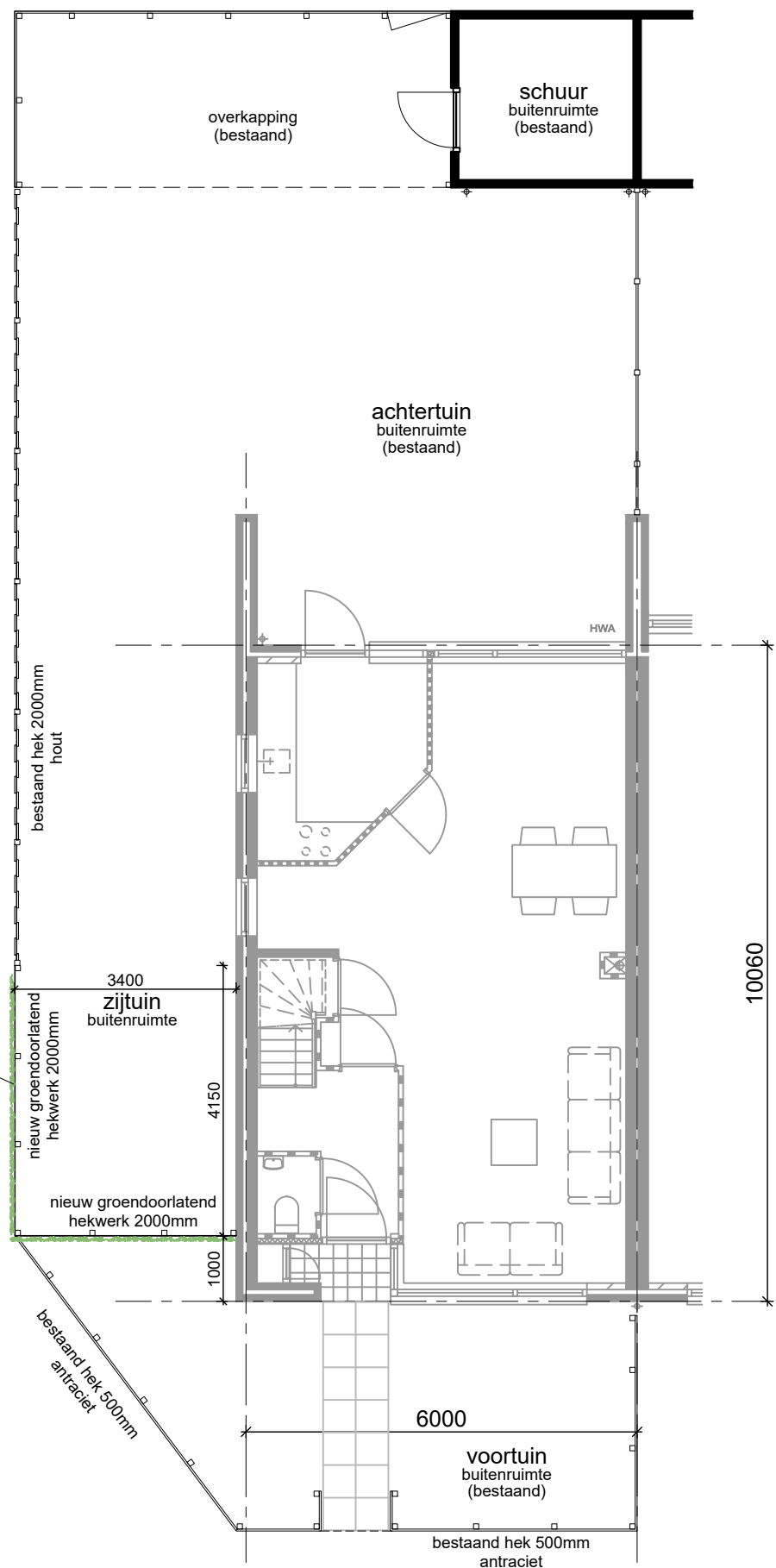
Begane grond nieuw schutting
