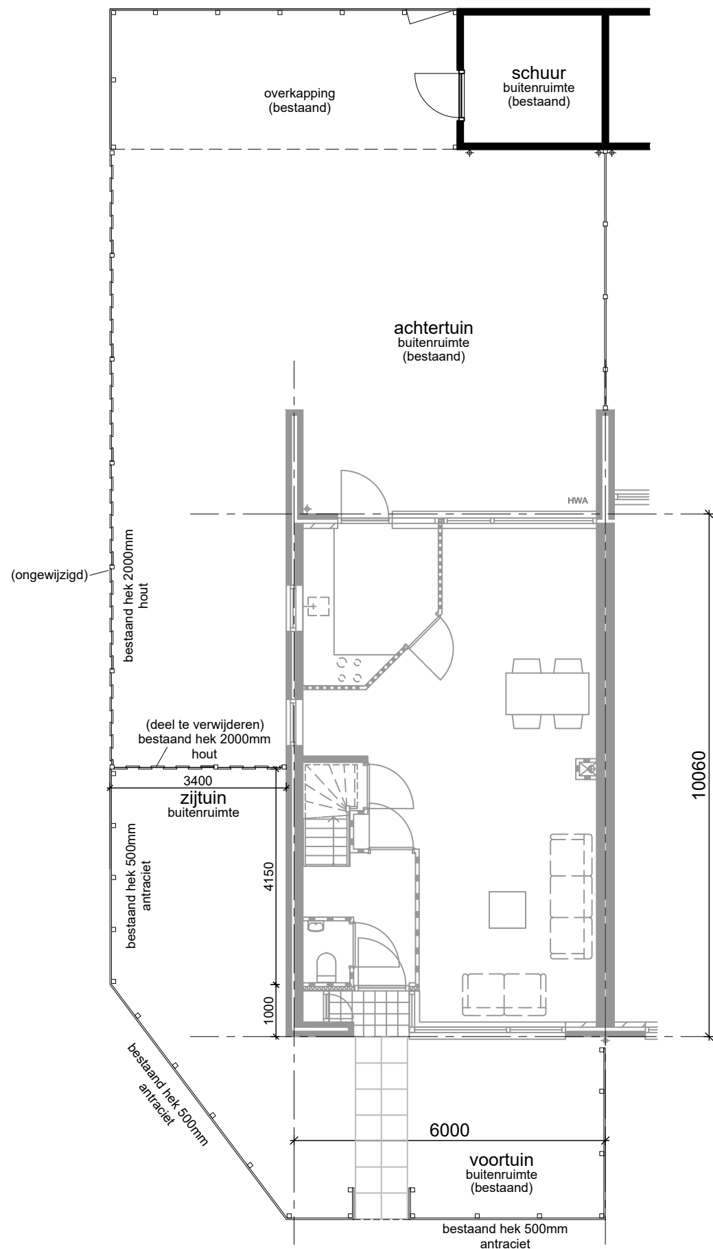
Begane grond bestaand schutting
