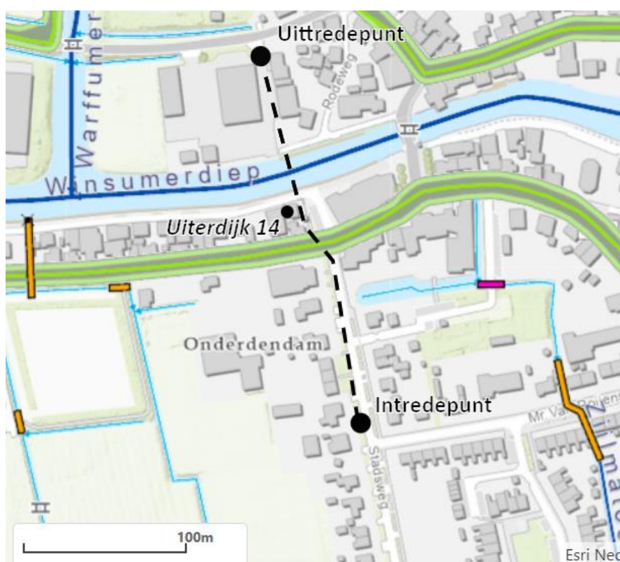
Figuur 1: Situatieschets traject gestuurde boring (stippellijn) ter hoogte van Uiterdijk 14 te Onderdendam (met groen is de regionale kering aangegeven)
