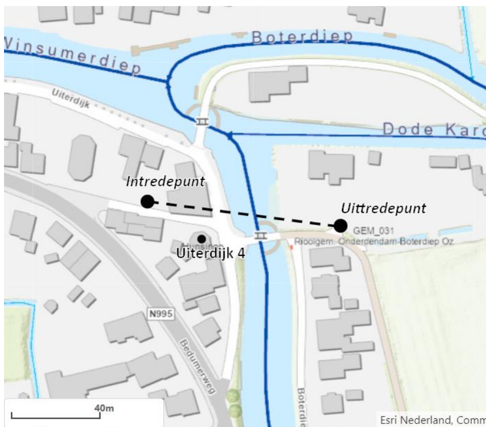
Figuur 1: Situatieschets traject gestuurde boring (stippellijn) ter hoogte van Uiterdijk 4 te Onderdendam
