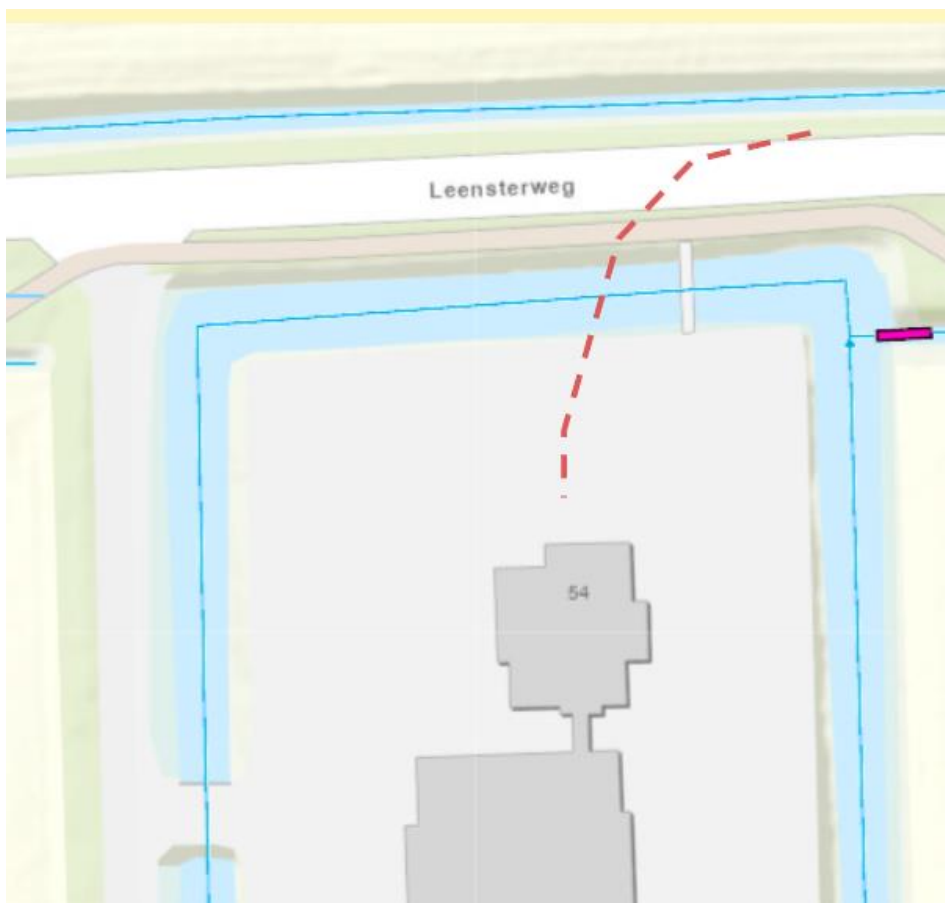
Figuur 4: Ingediende tekening 3, kruising (gestuurde boring) secundaire watgang.
