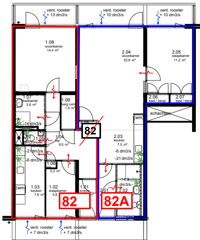
PLATTEGROND NIEUWE TOESTAND
