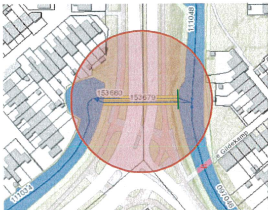
Figuur 2: Ingezoomd locatie bestaande duikers (rood) met de toekomstig kantelstuwen (groene streep).
