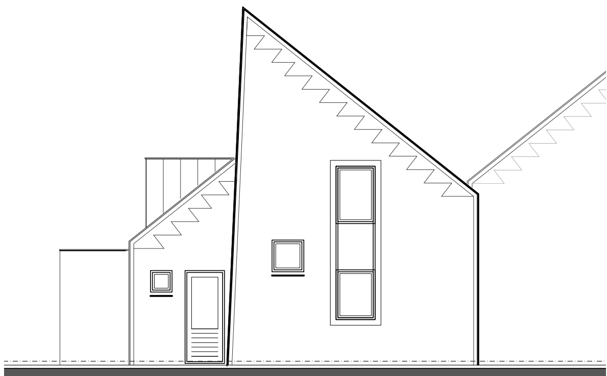
zuid-gevel
