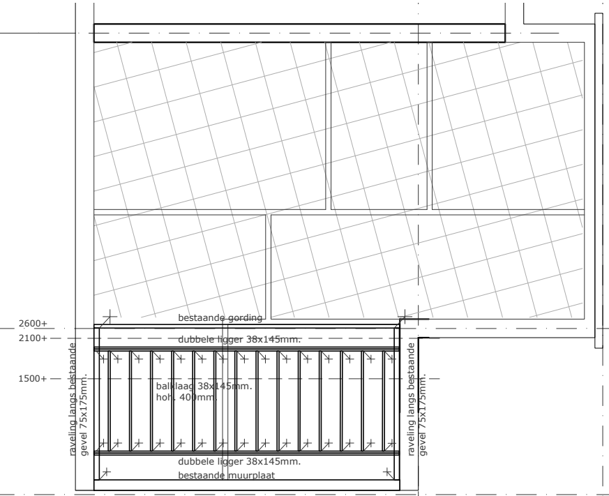
verdieping
