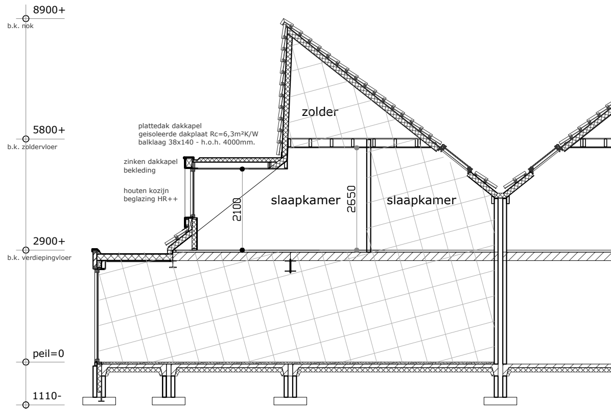
doorsnede
