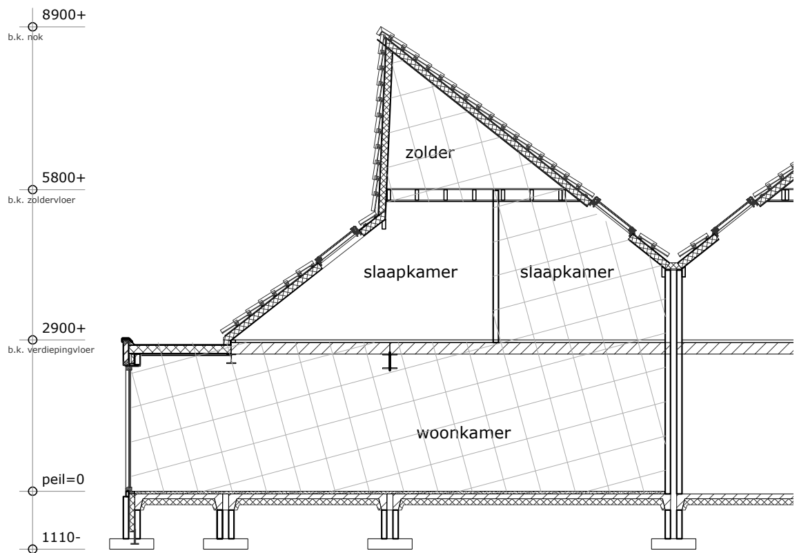
doorsnede
