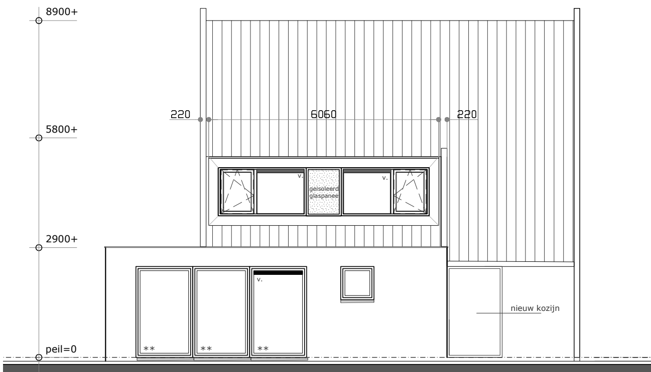
west-gevel
