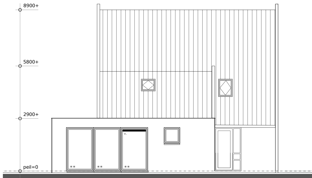
west-gevel
