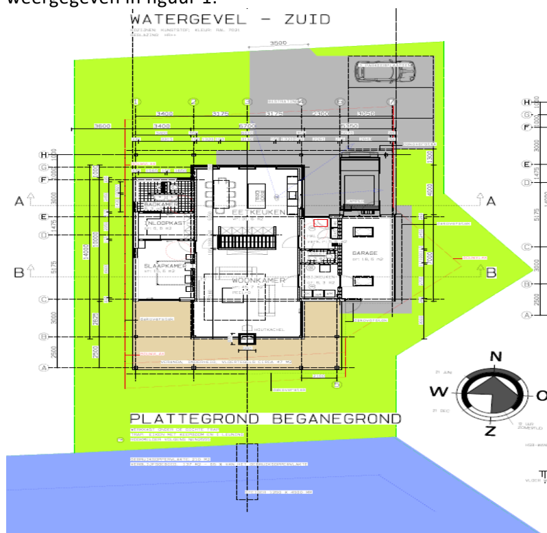
Figuur 1: De afbeelding toont de locatie van de aan te leggen steiger in het blauwe vlak.
