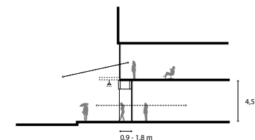
Ter plaatste van de entrees aan de kade worden setbacks van 0,9 - 1,8m tov de rooijlijn aangemoedigd
