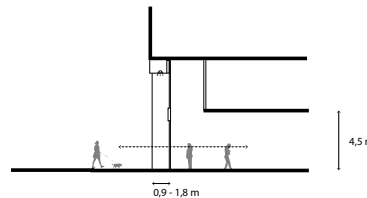
Entrees aan de greens zijn dubbelhoog en voorzien van een setback van 0,9 - 1,8 m tov de rooilijn
