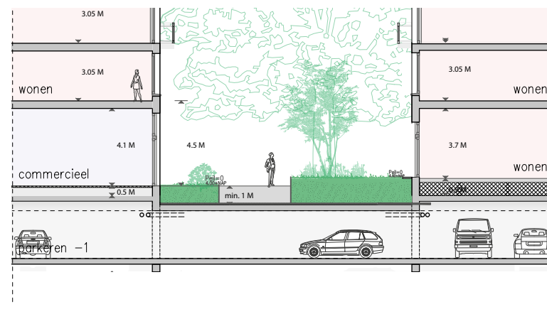
Maatvoering en uitgangspunten van de garage in relatie tot dekking in het maaiveld
