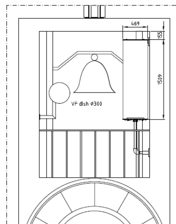
VOORAANZICHT NIEUW
