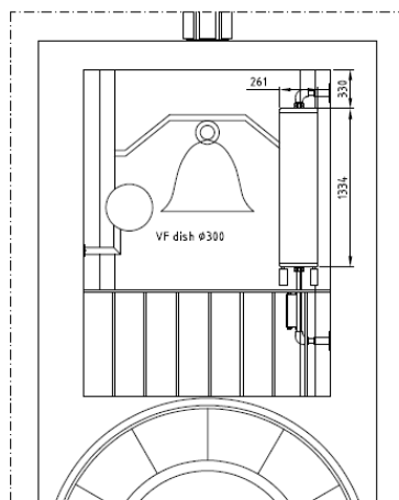
VOORAANZICHT BESTAAND
