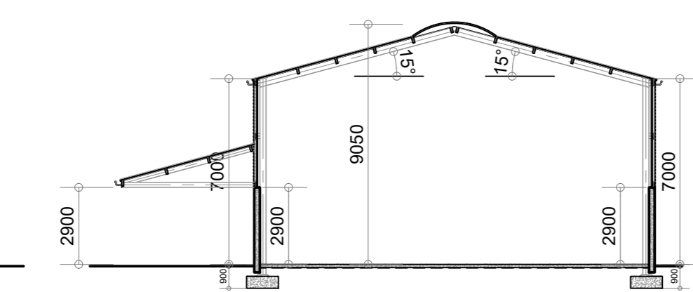
- Doorsnede A - A - gebouw 1 -
