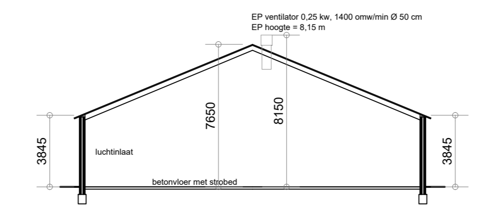
- Doorsnede B - B - gebouw 2 -
