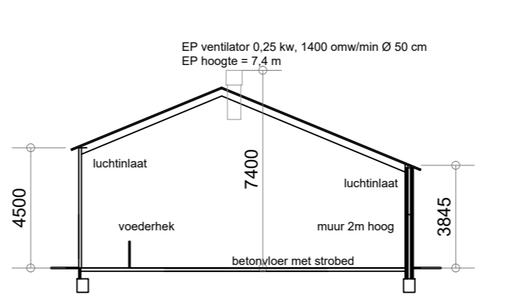
- Doorsnede C - C - gebouw 2 -
