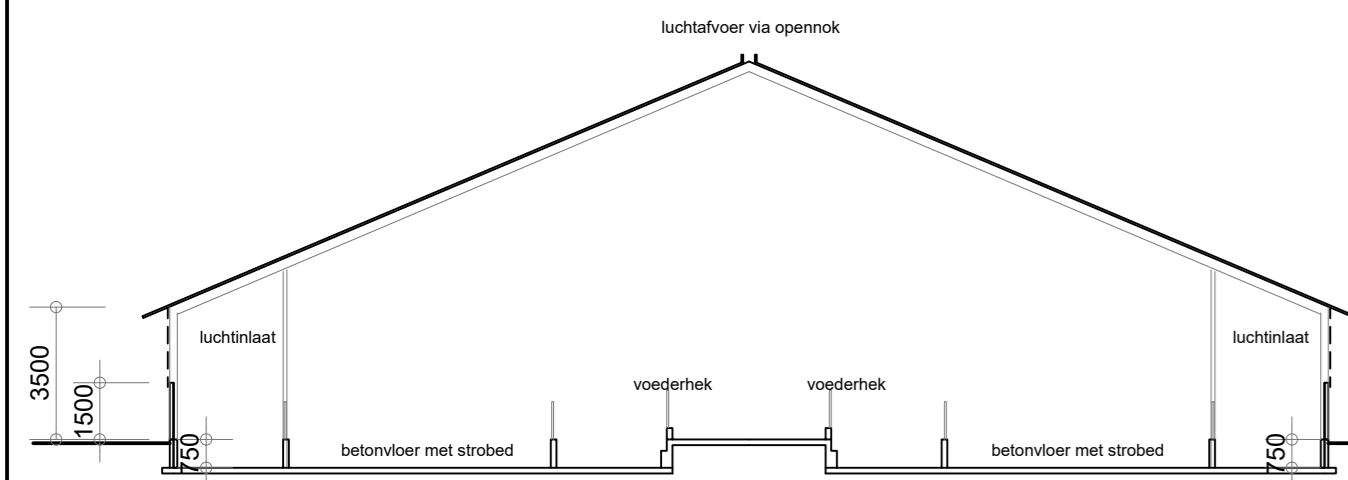
- Doorsnede D - D - gebouw 5 -
