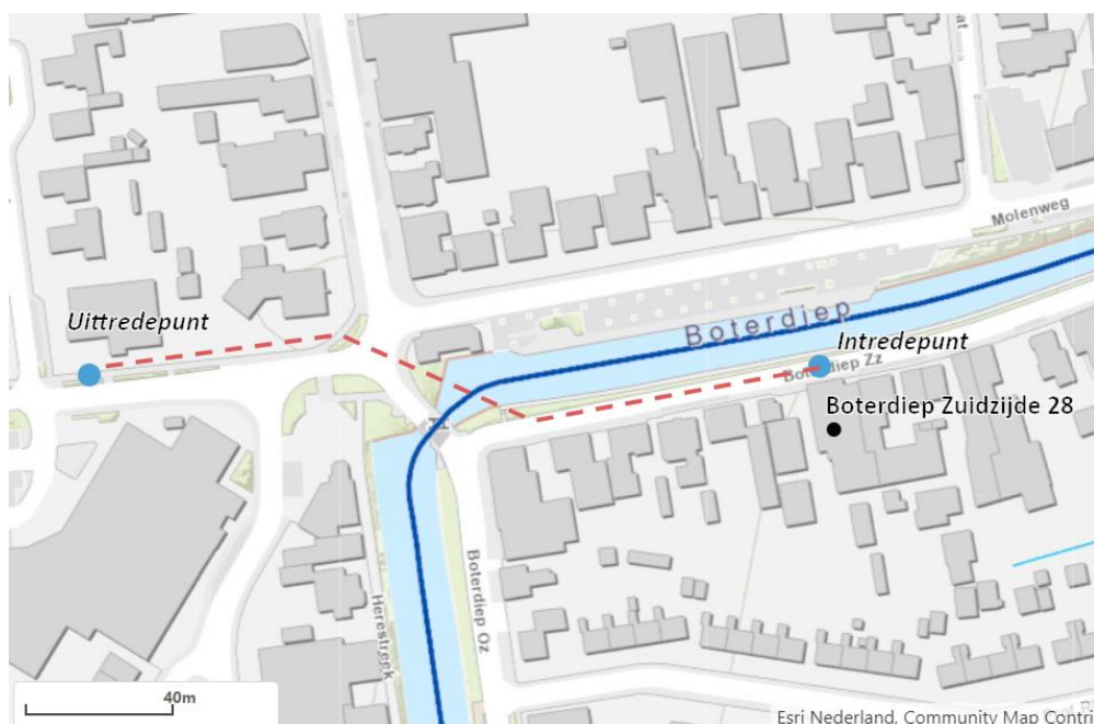
Figuur 1: Situatieschets traject gestuurde boring (rode stippellijn) ter hoogte van Boterdiep Zuidzijde 28 te Bedum
