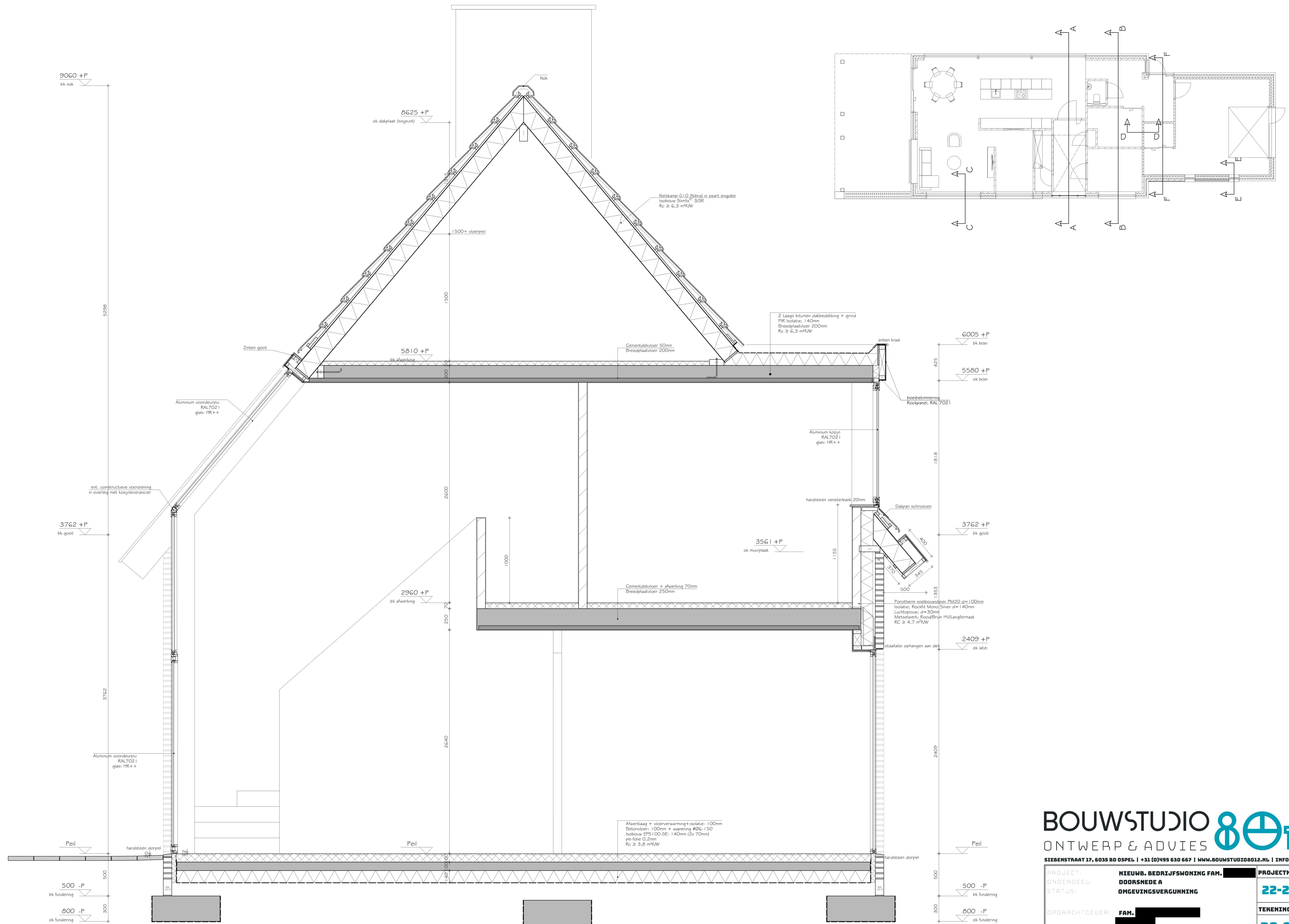
DOORSNEDE A
