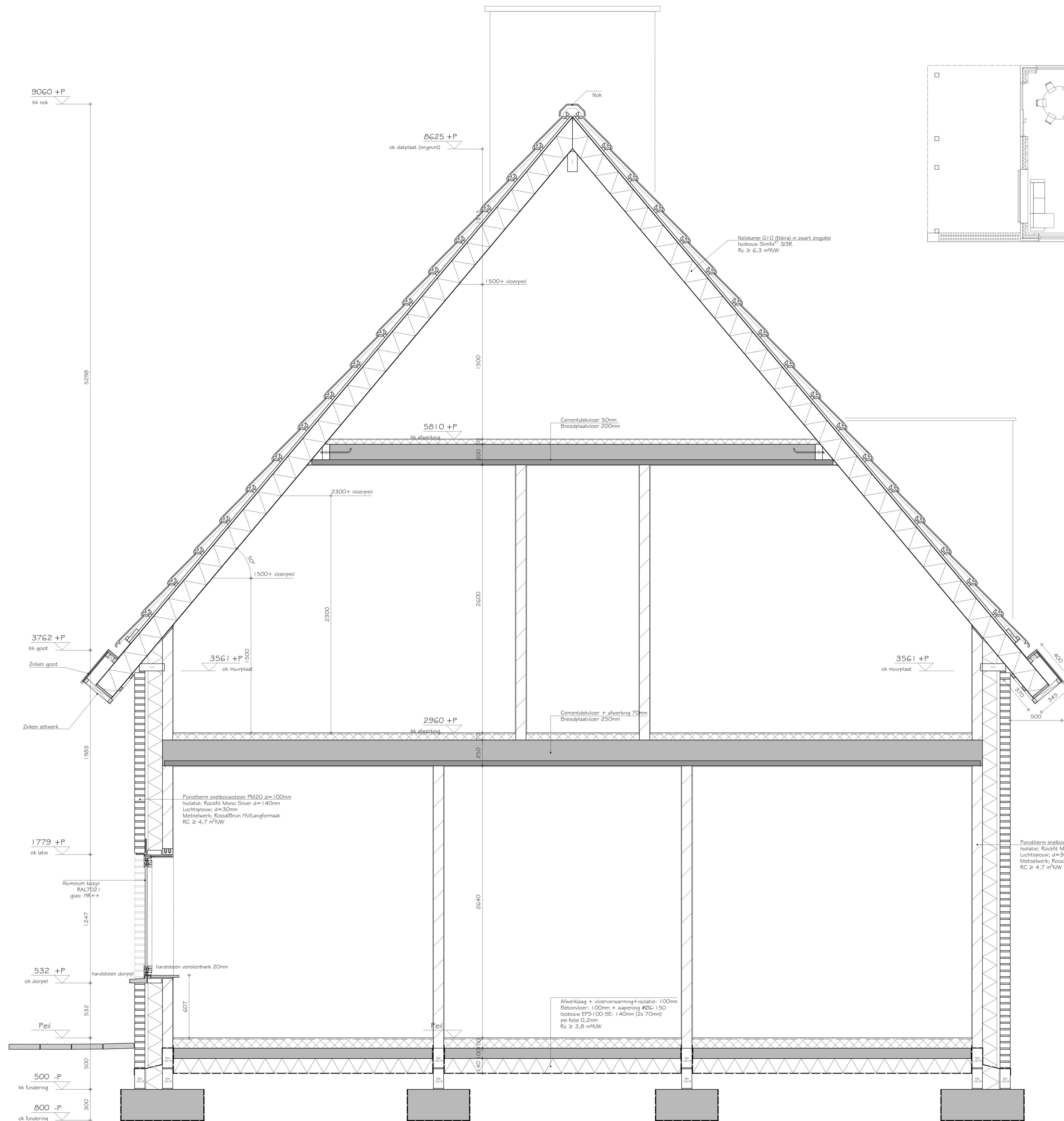
DOORSNEDE B
