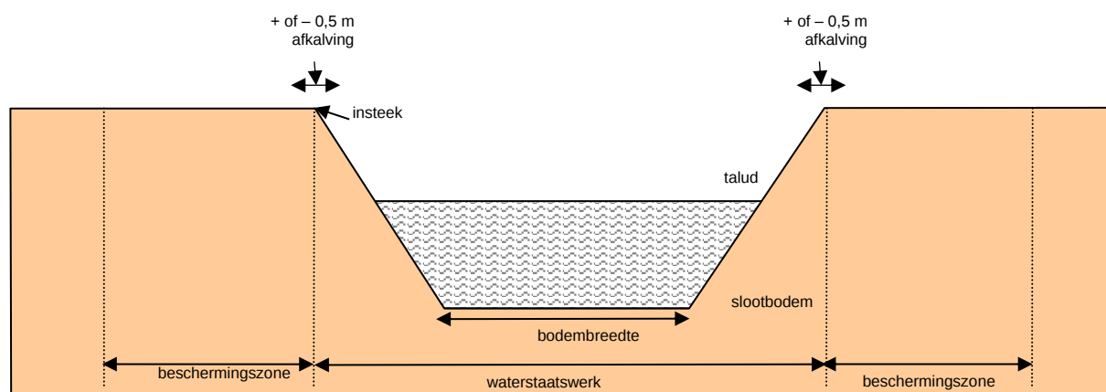
Figuur 5 Bandbreedte afkalving
