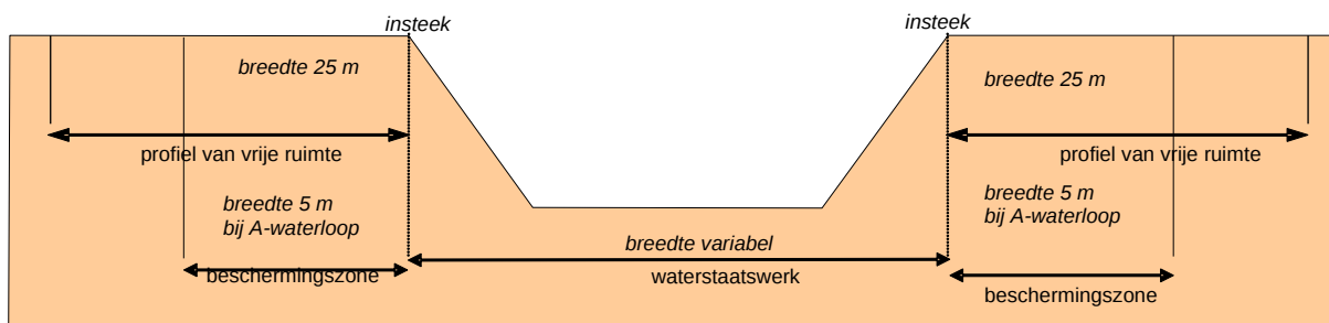
Figuur 5 Beschermingszones en profiel van vrije ruimte
