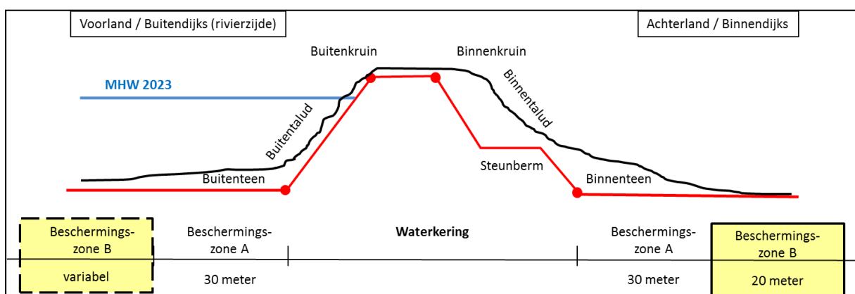
Figuur 4.3: Beschermingszone B
