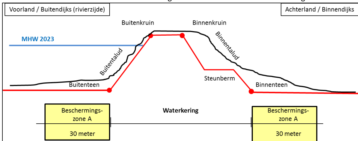
Figuur 4.2: Ligging beschermingszone A bij primaire waterkeringen
