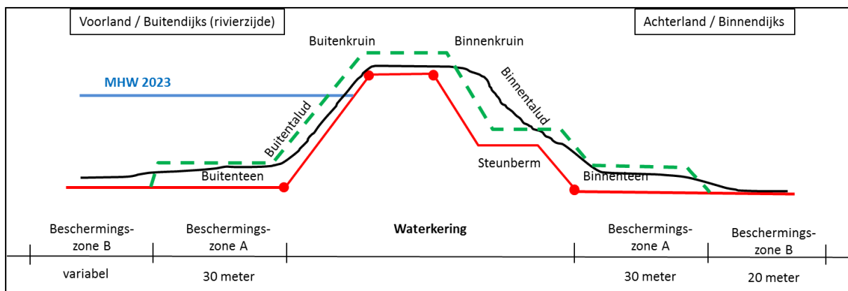
Figuur 4.4: profiel van vrije ruimte (groene stippellijn)
