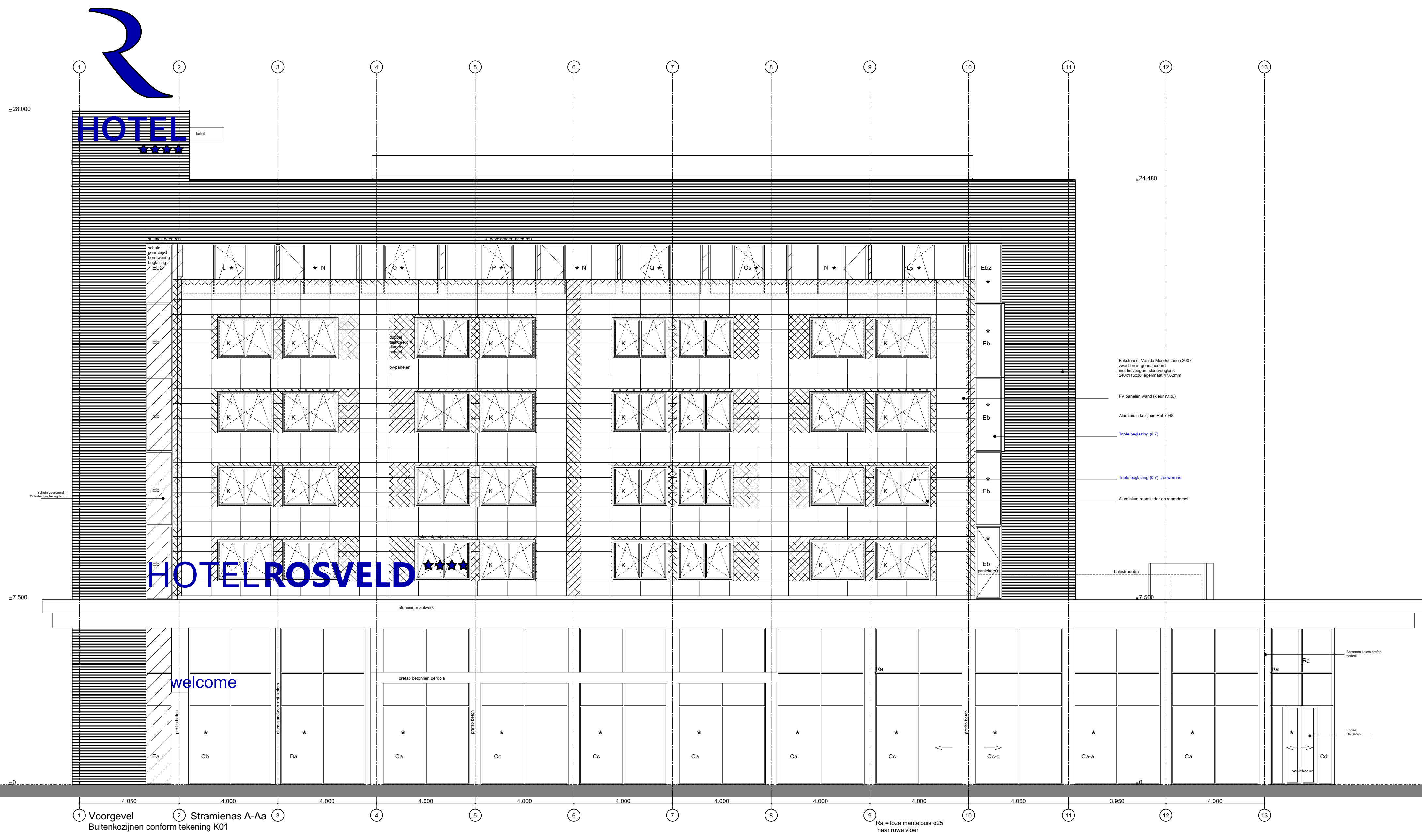
Voorgevel Stramienas A-Aa Buitenkozijnen conform tekening K01
