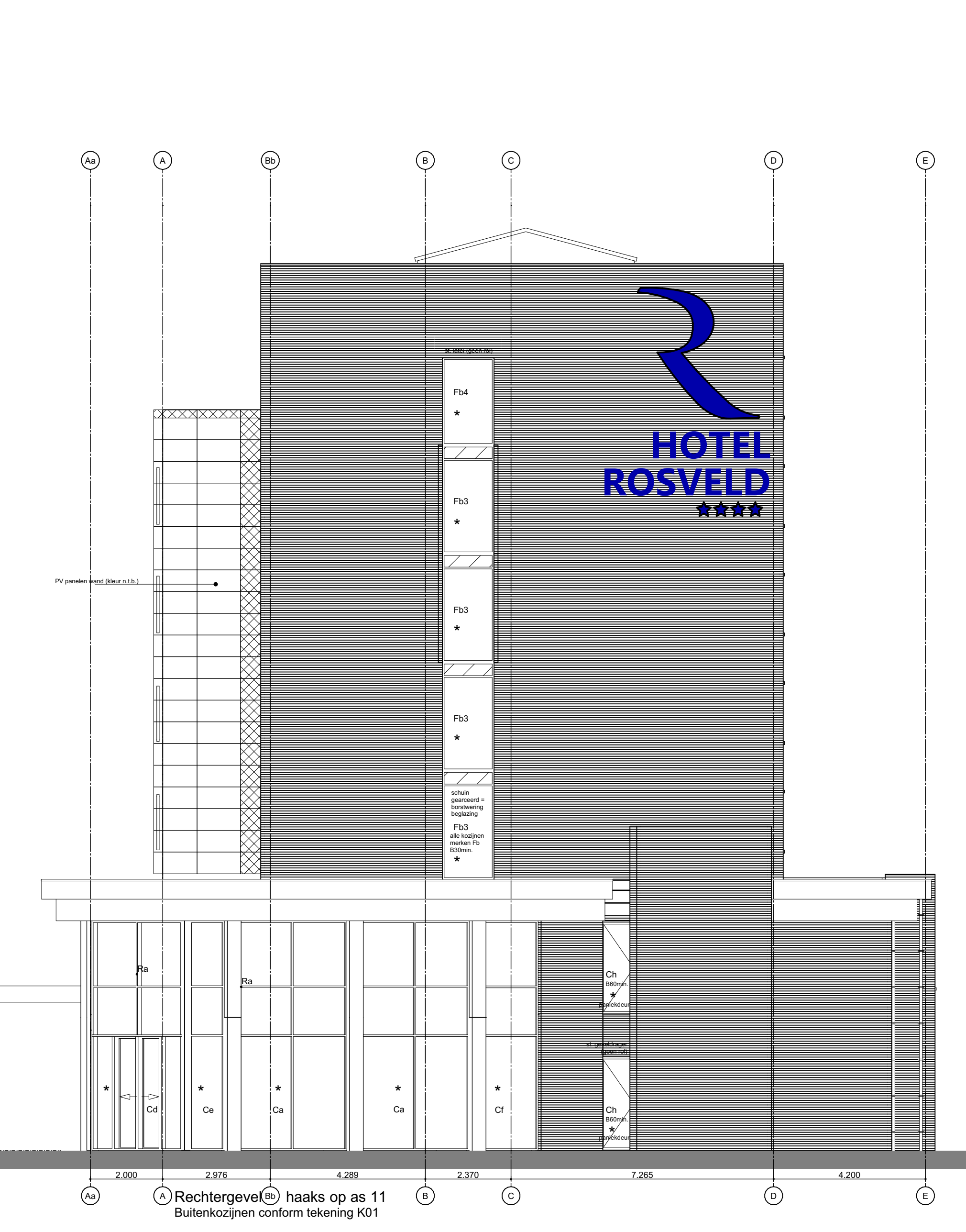
Rechtergevel haaks op as 11 Buitenkozijnen conform tekening K01
