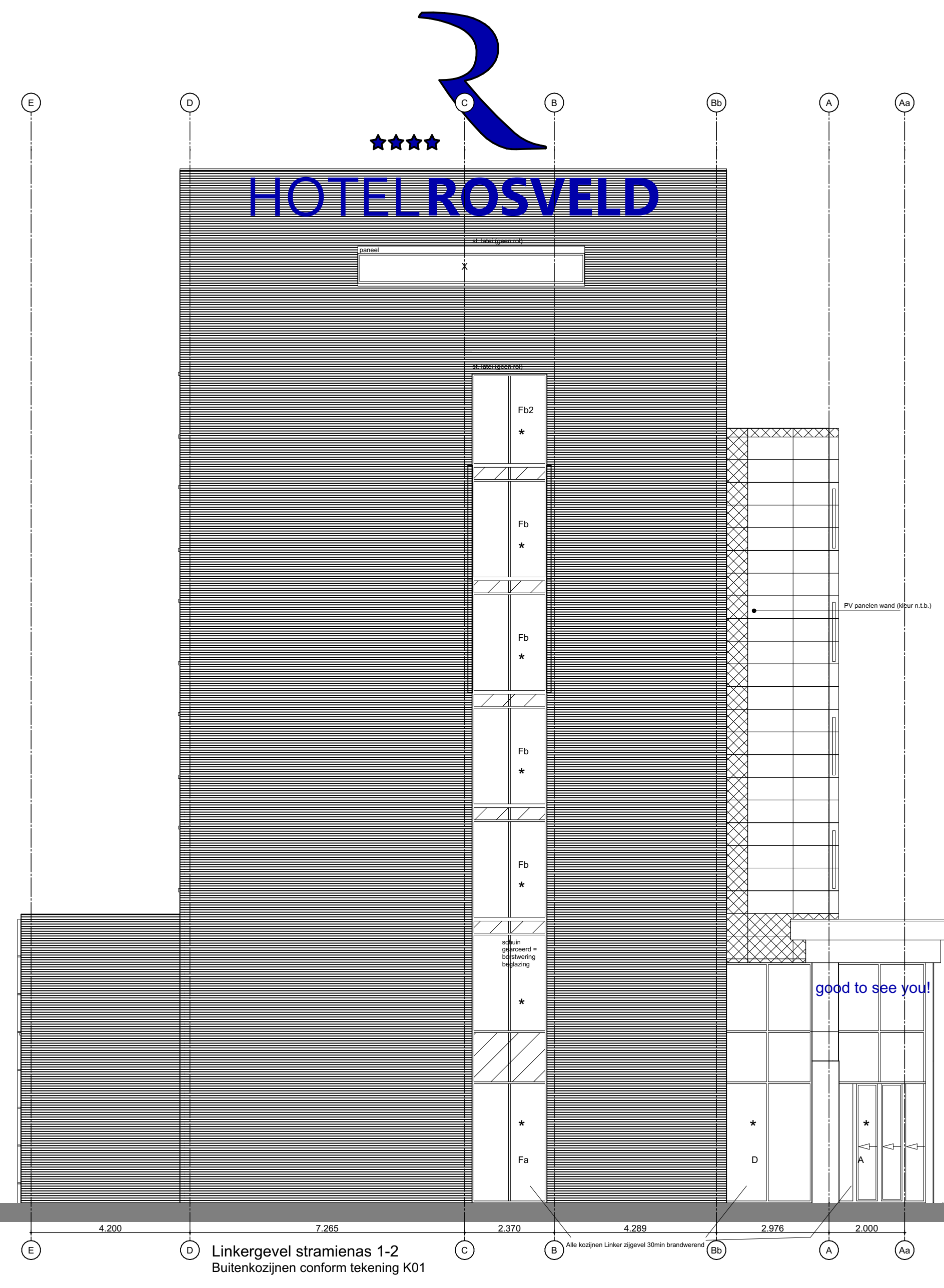
Linkergevel stramienas 1-2 Buitenkozijnen conform tekening K01
