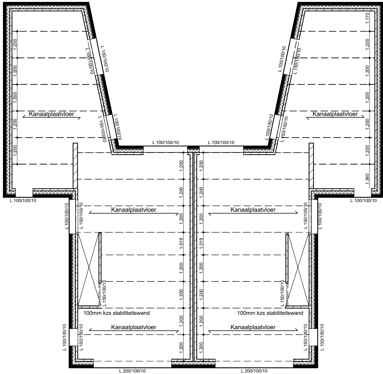
0. 1e verdieping 1:100
