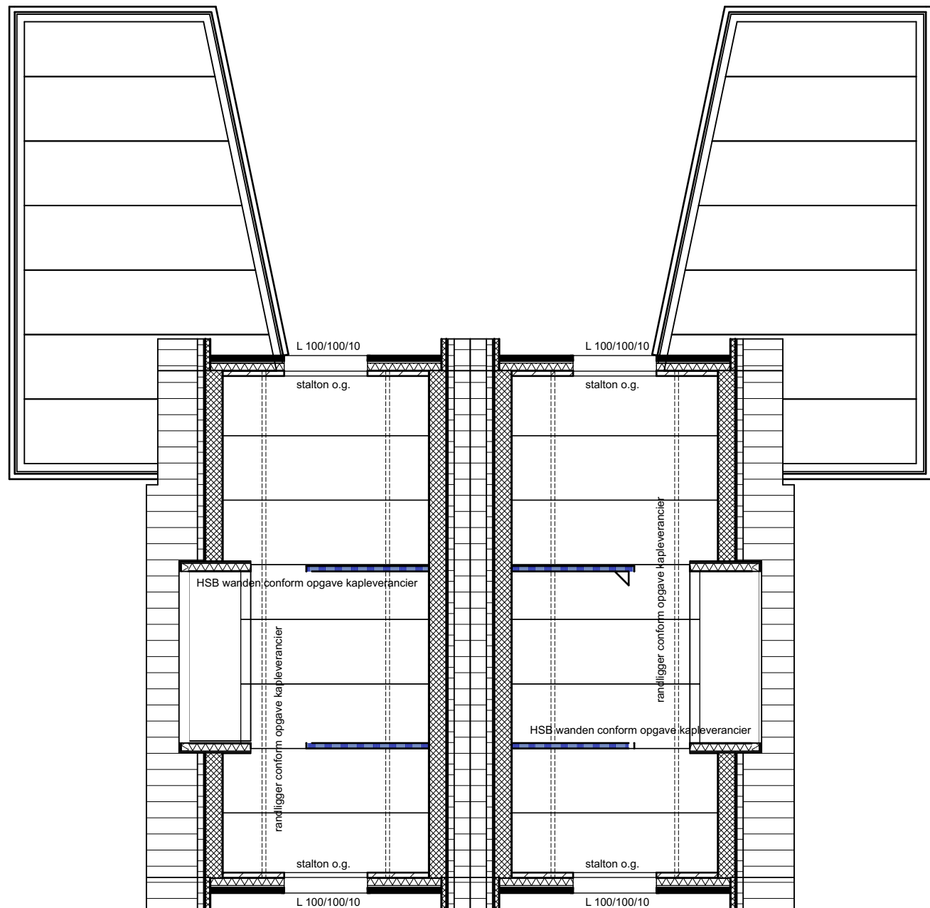
1. kap 1:100
