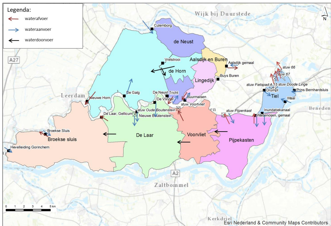
Afbeelding 2.7 Schematische tekening watersysteem Tielerwaard en Lek en Linge
