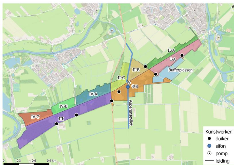
Afbeelding 2.1 Ligging secties en beschreven kunstwerken binnen Nieuwe Zuiderlingedijk inclusief Asperensevliet
