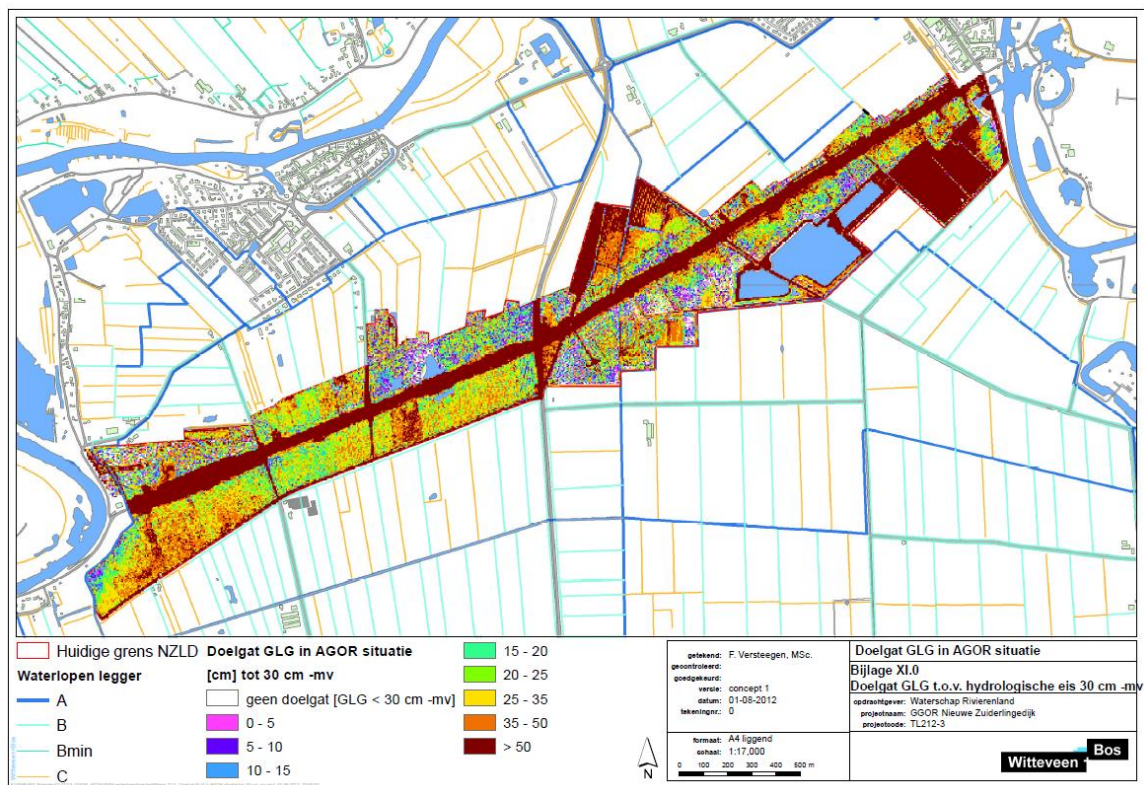
Afbeelding 7.2 Doelgat-kaart GLG Nieuwe Zuiderlingedijk
