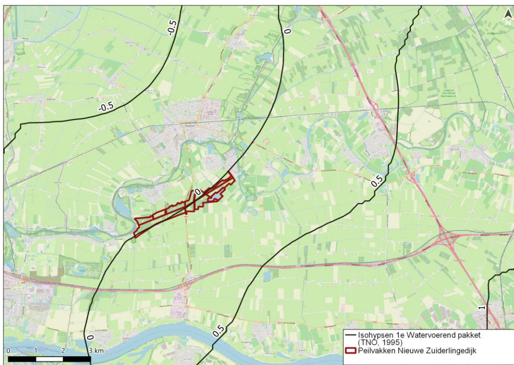
Afbeelding 2.6 Isohypsenaart stijghoogte in het eerste watervoerende pakket in de omgeving van de Nieuwe Zuiderlingedijk (rood omkaderd)
