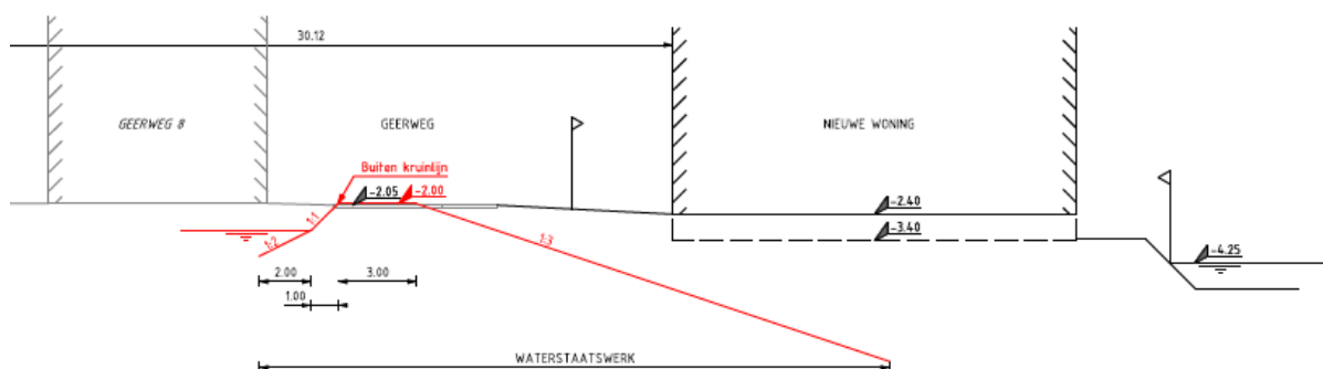
Tekening "file :...\Geerweg 9 Nootdorp_29-04-2022.dgn", ongenummerd, d.d. 29 april 2022, behorend bij de aanvraag.
