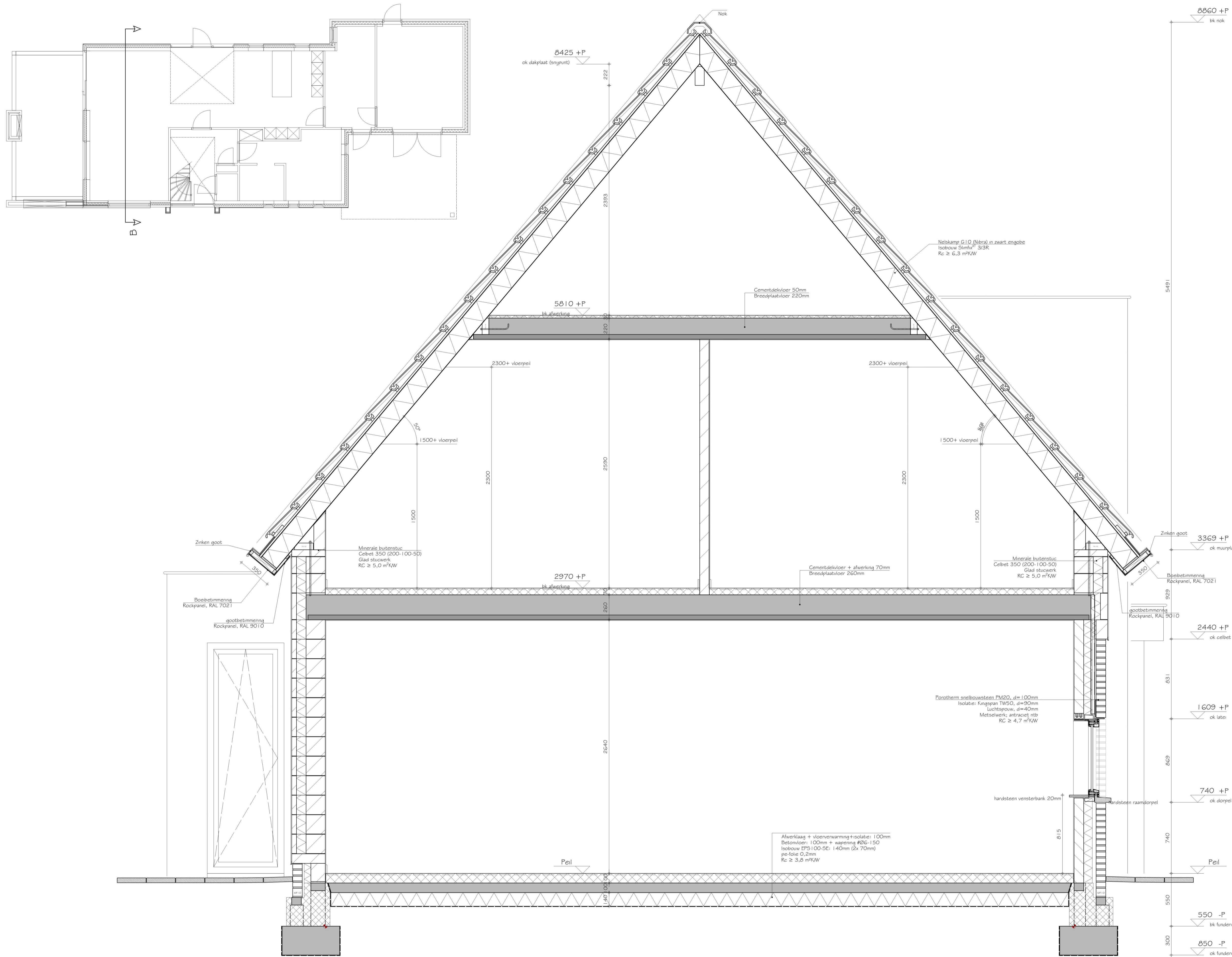
SNEDE B-B
