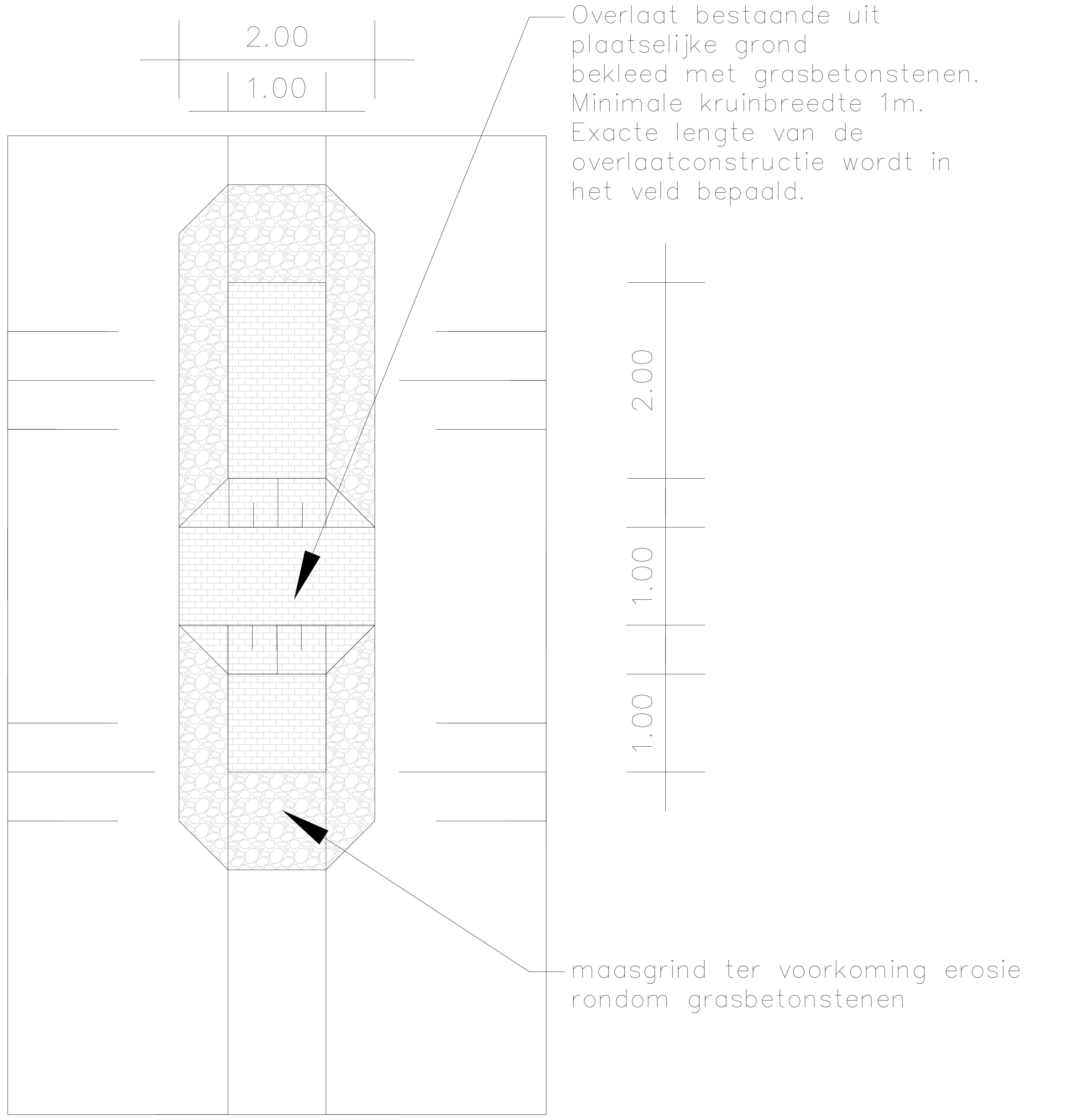
Bovenaanzicht 1:20
