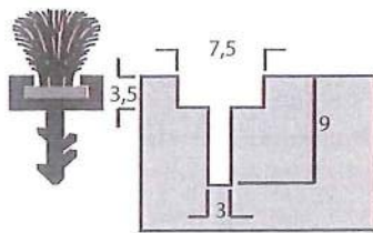
Borstelhouder
