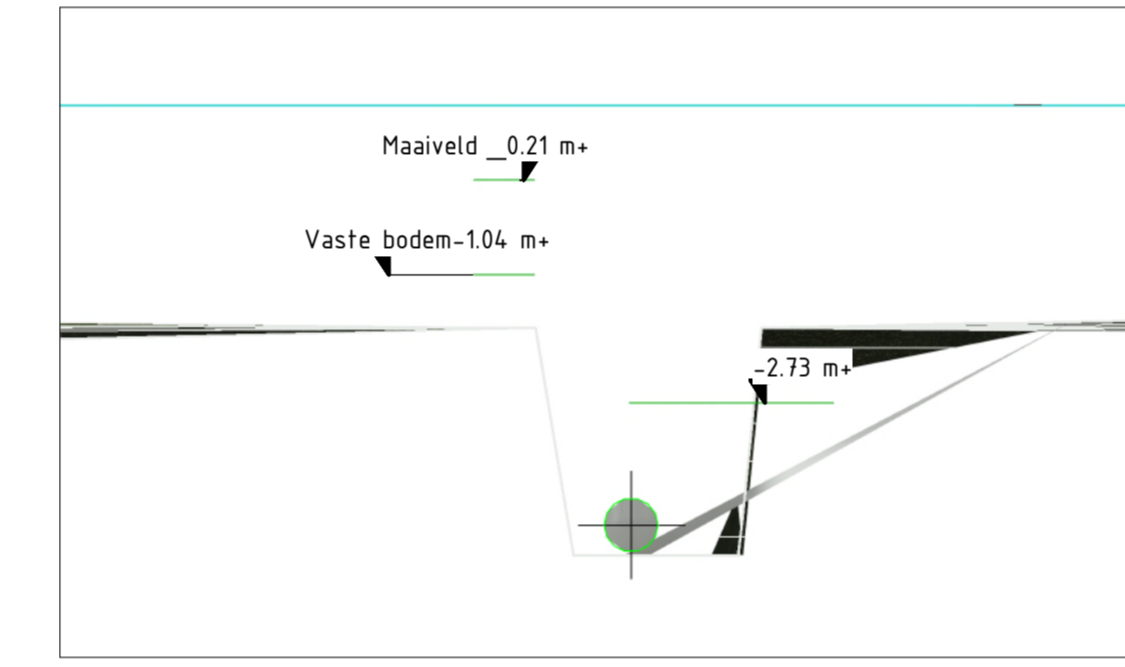
Doorsnede 4 - doorsnede Grote Wiel schaal 1: 100
