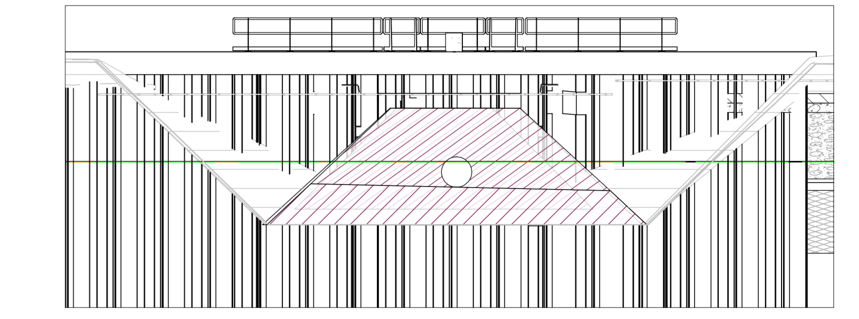
Doorsnede 2 - dijk doorkruising schaal 1: 100
