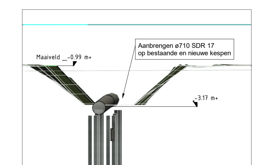
Doorsnede 6 - bestaand/ nieuw trace schaal 1: 100
