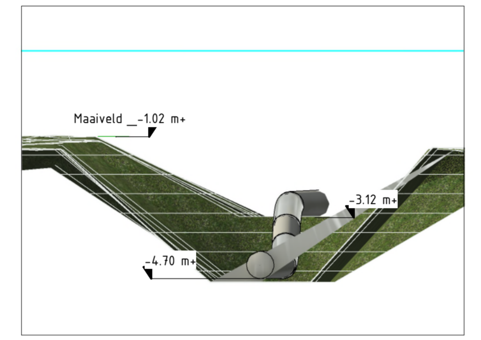
Doorsnede 5 - ontgraving t.p.v. zinker schaal 1: 100
