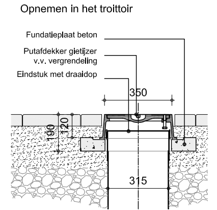
DETAIL 3 DOORSPIJTPUT RINGLEIDING
