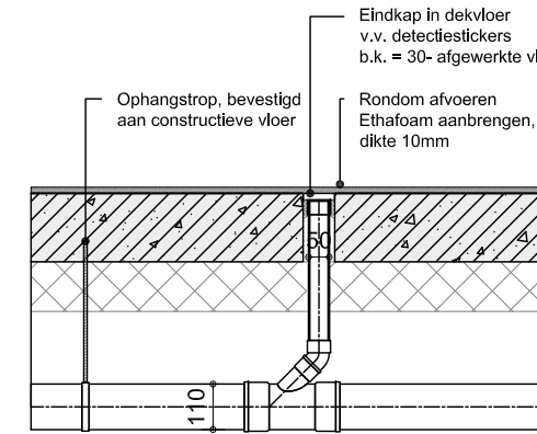
DETAIL 2 T-STUK RINGLEIDING ONDER STELLINGEN
