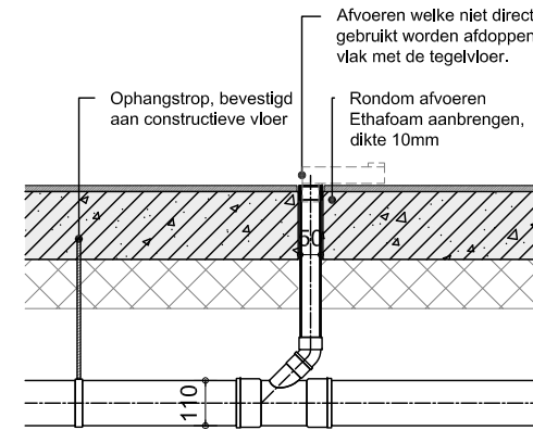
DETAIL 1 T-STUK RINGLEIDING ONDER KOELINGEN
