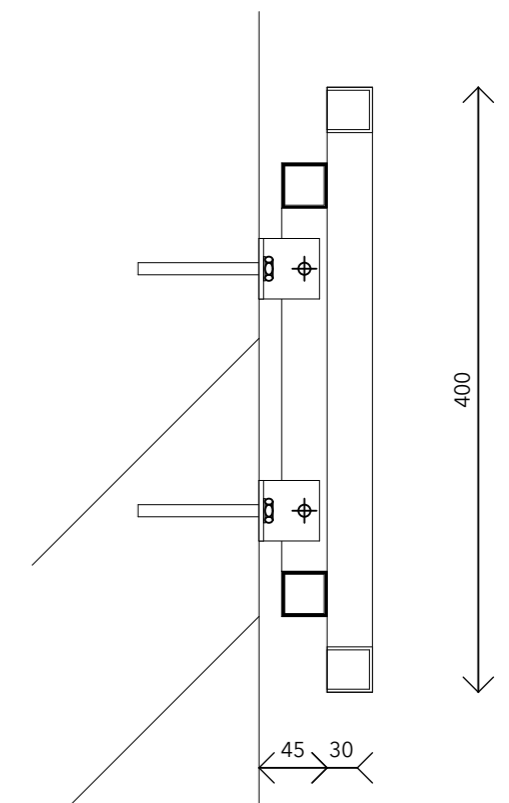
principe detail bevestiging 1:5
