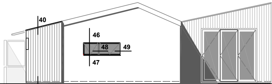
zuidgevel
