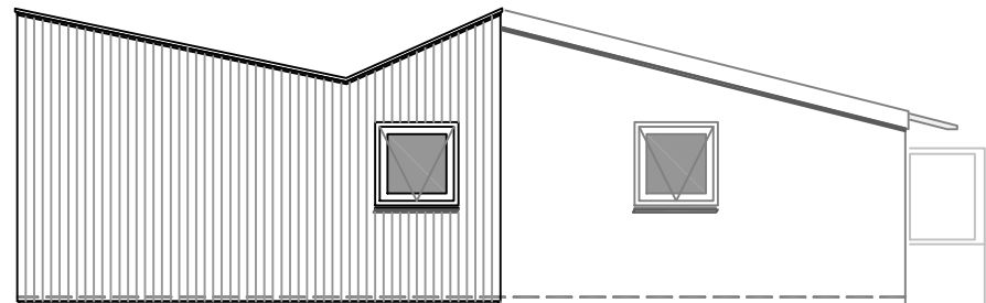
noordgevel
