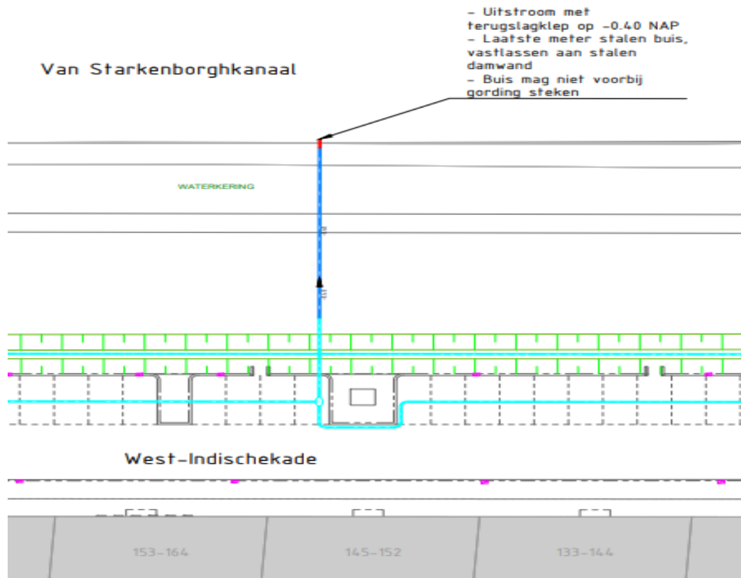
Figuur 2: Locatie gewenste uitstroomvoorziening, wadi in groen.
