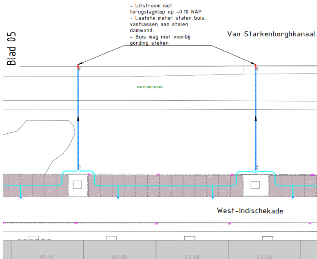
Figuur 3: Locaties gewenste uitstroomvoorzieningen
