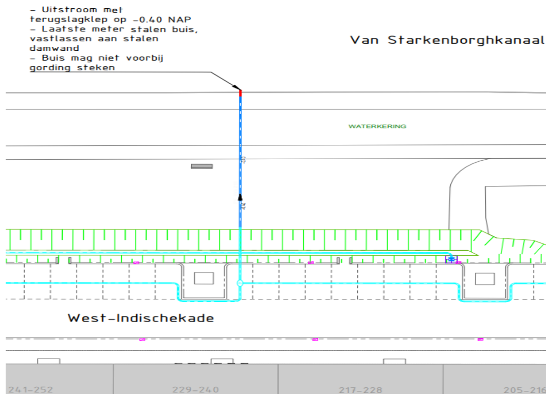
Figuur 1: Locatie gewenste uitstroomvoorziening, wadi in groen.
