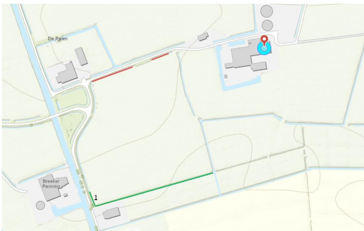
Figuur 1: Locatie van werkzaamheden. Rode lijnen geven te dempen watergang weer. Groene lijnen geven te verbreden watergangen weer.
