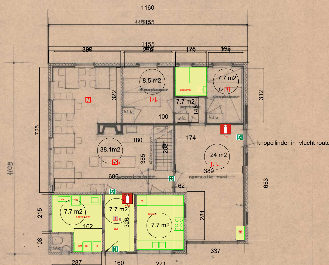
begane grond
