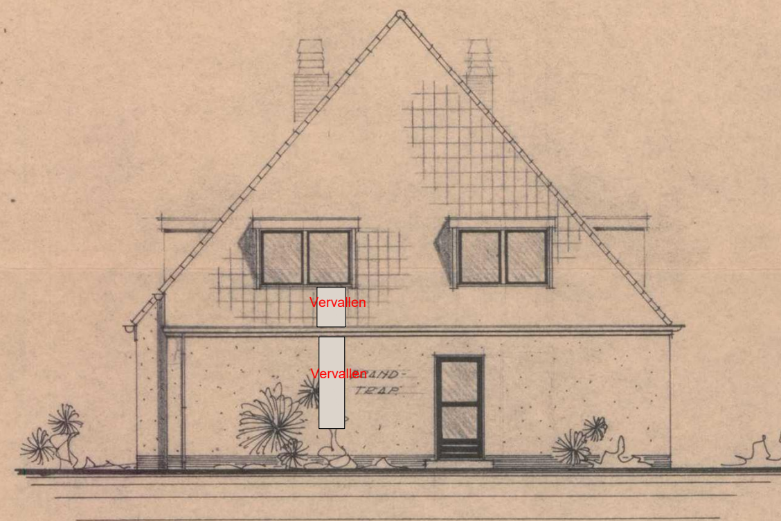
noordgevel
