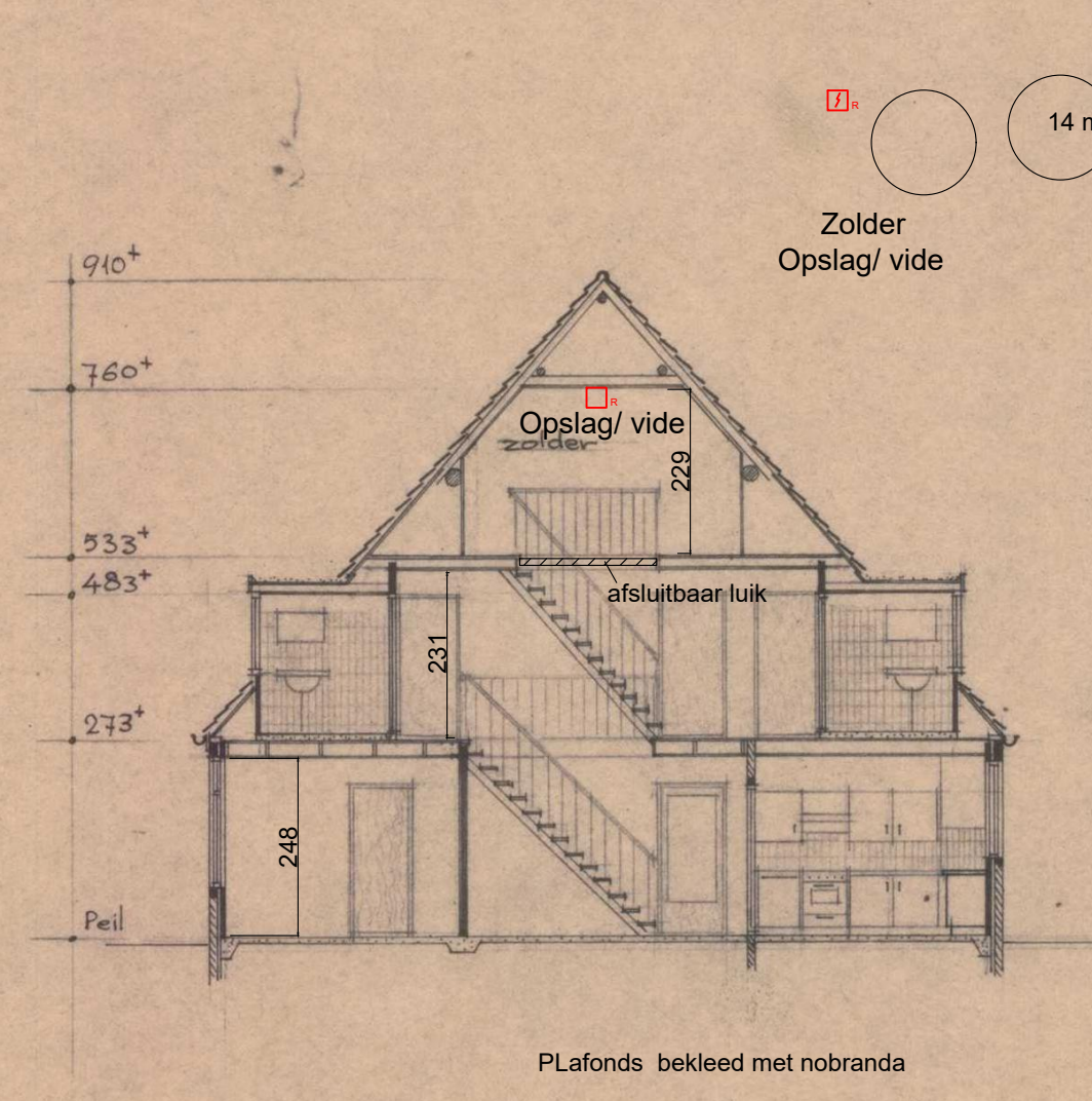
doorsnede
