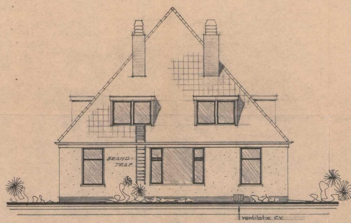
zuidgevel
