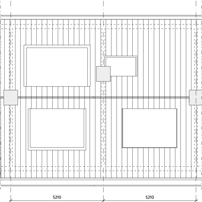
80 82 Dakaanzicht - bestaand
