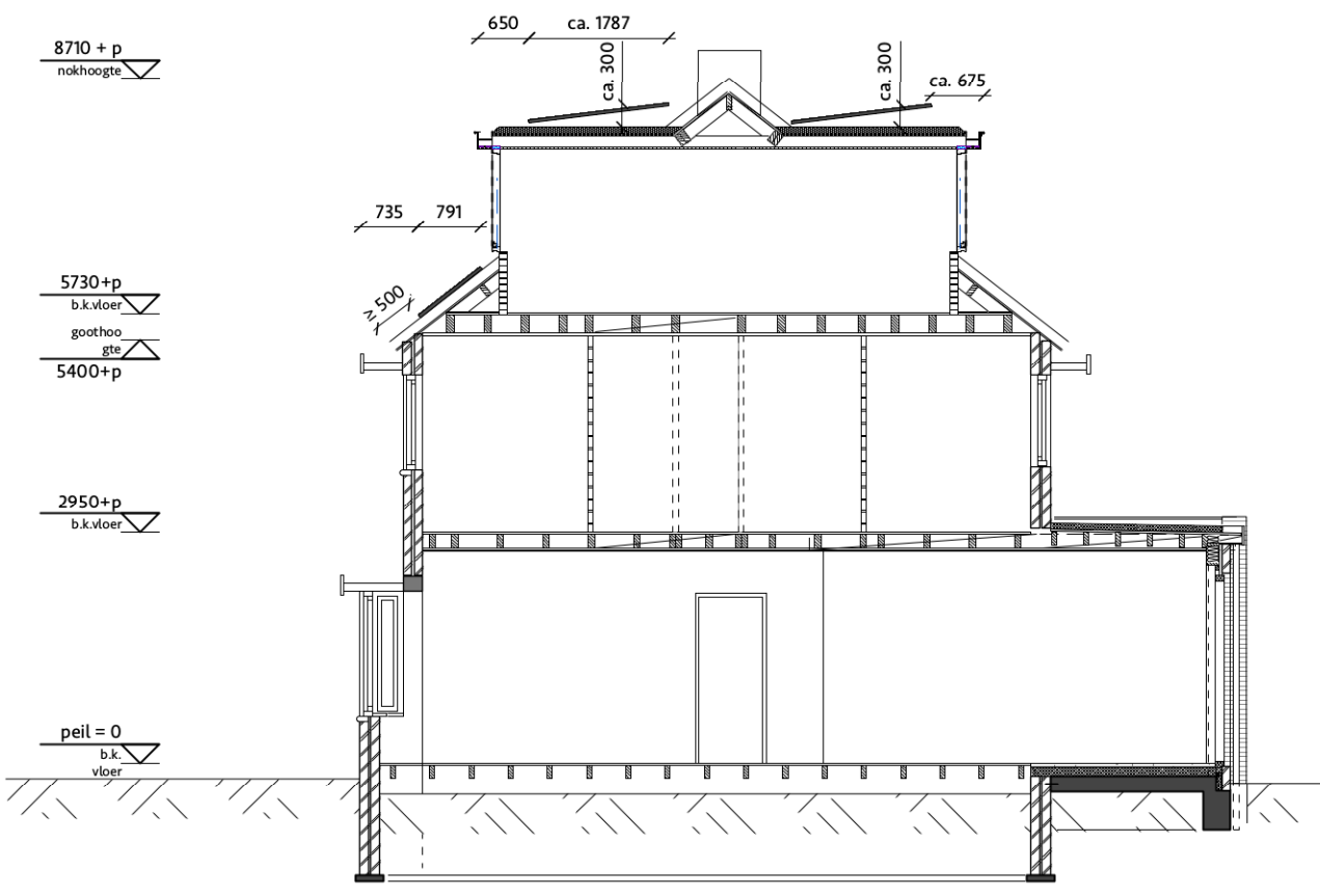
Doorsnede - gewijzigd
