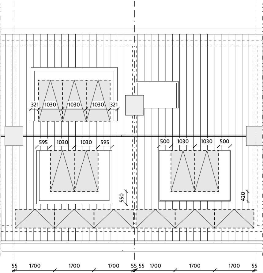
80 82 Dakaanzicht - gewijzigd
