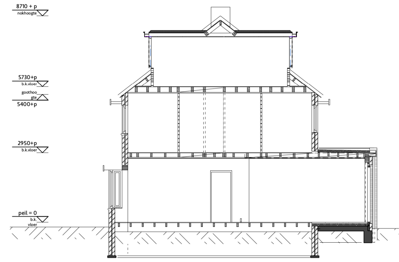
Doorsnede - bestaand
